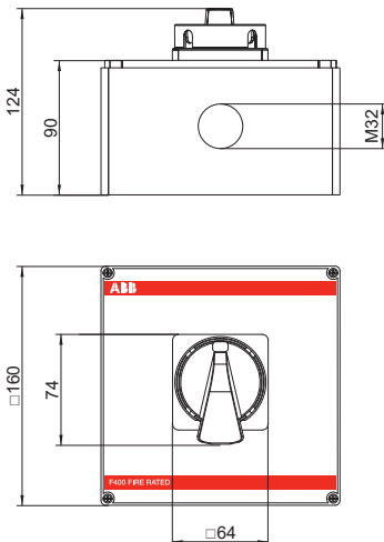
Box size OKA 40_F4_ F-400 40A
