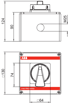
Box size OKA 25_F4_ F-400 25A
