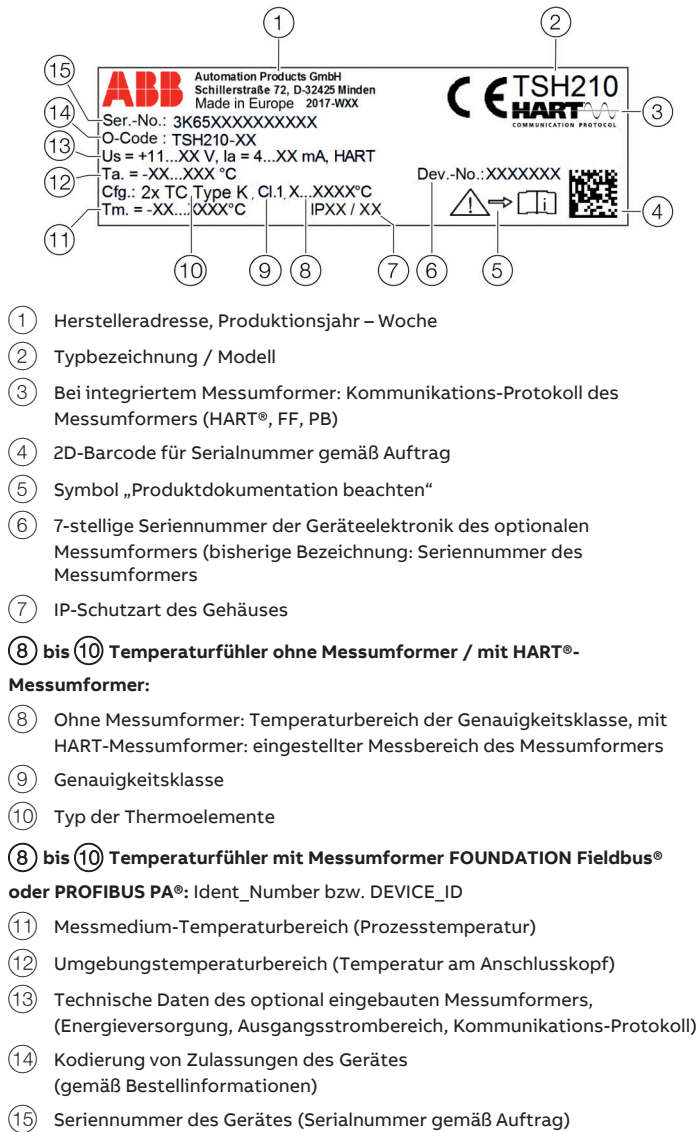
Abbildung 1: Typenschild (Beispiel)
