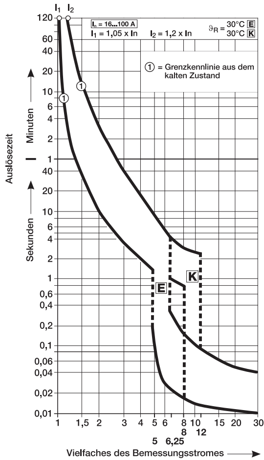
Auslösekurve 16 ... 100 A
