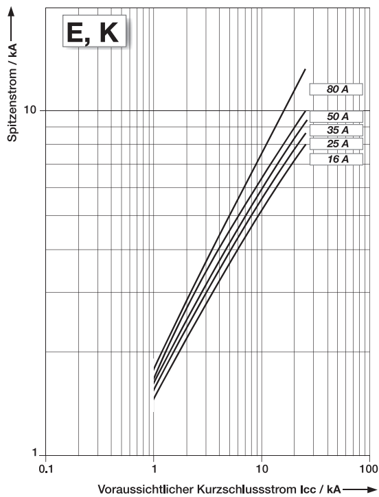
Diagramm der Durchlasswerte I_p 16...100 A
