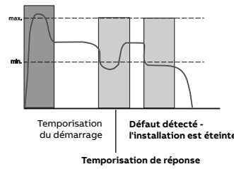
Protection contre la marche à sec
