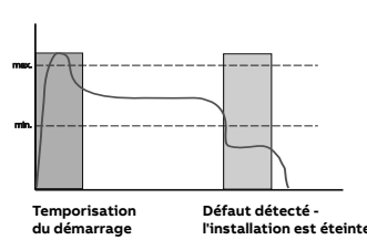
Surveillance du facteur de puissance
