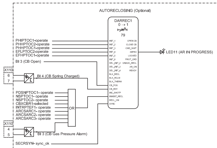
Figure 89: Autoreclosing
