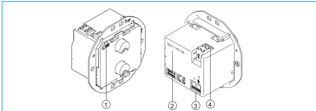
Abb. 2: Geräteübersicht Sensor/Schaltaktor 1/1-fach und 2/1-fach
