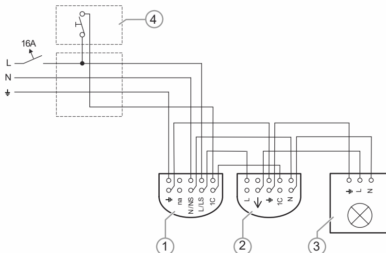
Afb. 48: Schakelvoorbeelden: gang (hoofdpost/nevenpost) lichtsturing met nevenpostingang
