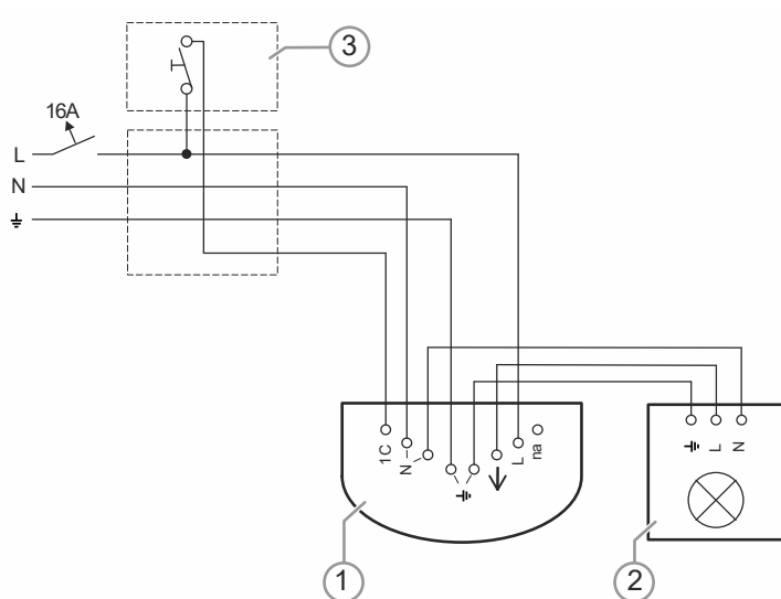
Afb. 24: Schakelvoorbeelden: individueel kantoor lichtregeling met nevenpostingang
