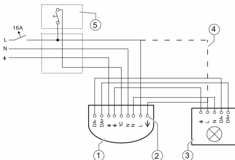
Afb. 38: Schakelvoorbeelden: eenvoudig toilettensysteem DALI-lichtsturing met nevenpostingang
