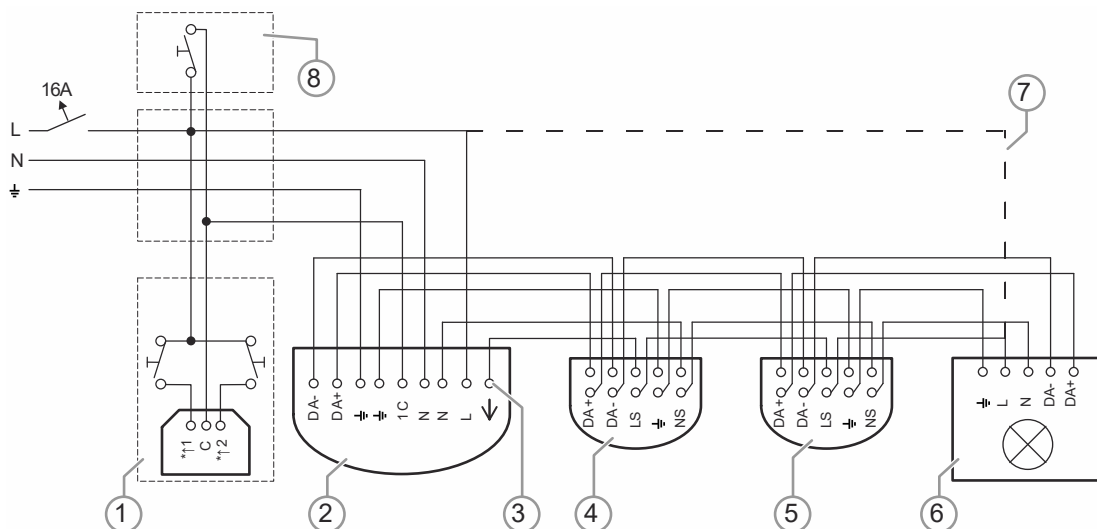
Afb. 36: Schakelvoorbeelden: kantoortuin (hoofdpost/nevenpost) DALI-lichtsturing met nevenpostingang
