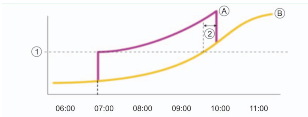
Afb. 43: Regeling bij functie constantlichtschakelaar
