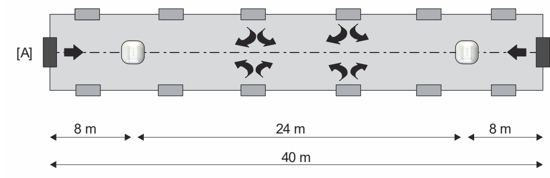
Afb. 46: Toepassingsvoorbeeld: doodlopende gang met twee deuren (brandcompartiment)
