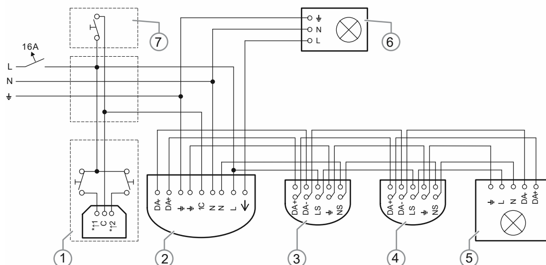
Afb. 31: Schakelvoorbeelden: klaslokaal lichtsturing DALI met
