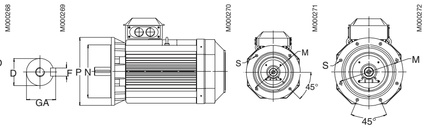
Flange mounted motor IM 3001, B5
