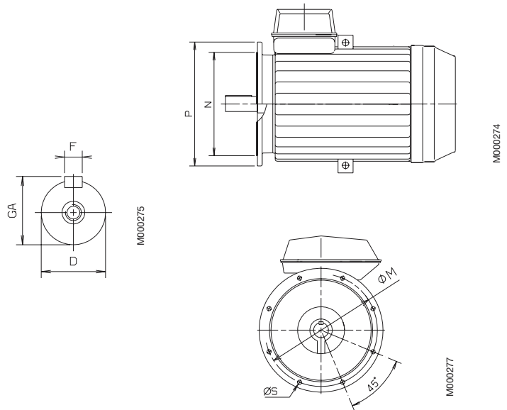
Flange mounted motor IM 3001, B5
