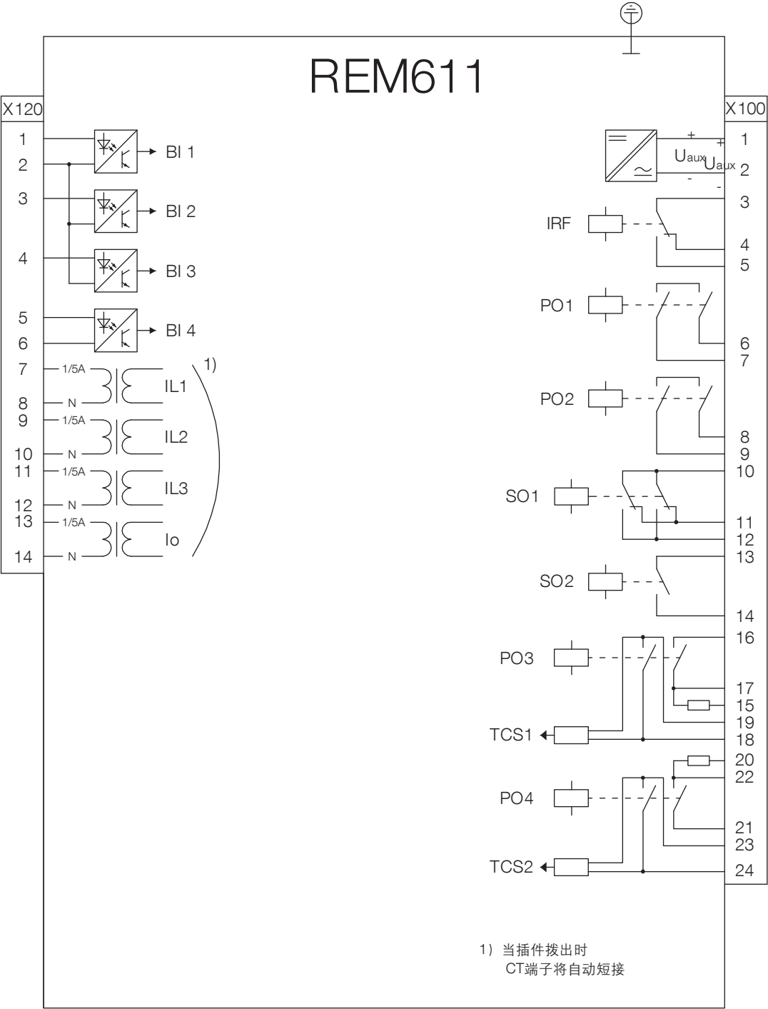
图10. 标准配置A接线图
