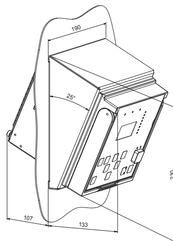
图8：倾斜25°的半嵌入式安装
