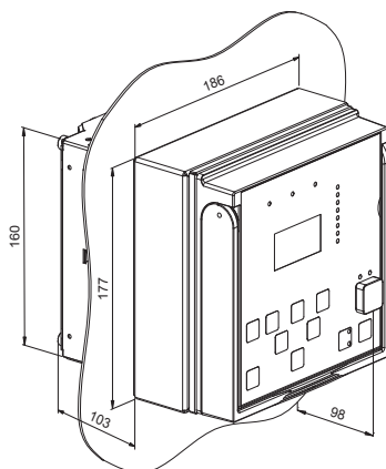
图 7：半嵌入式安装
