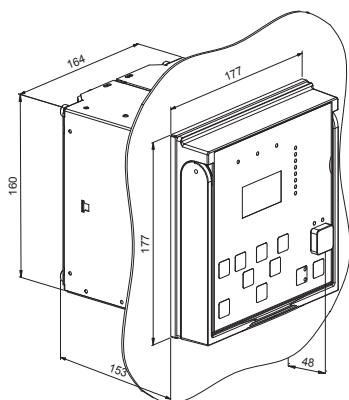
图 6：嵌入式安装
