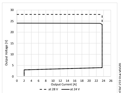
CP-S.1 24/20.0
