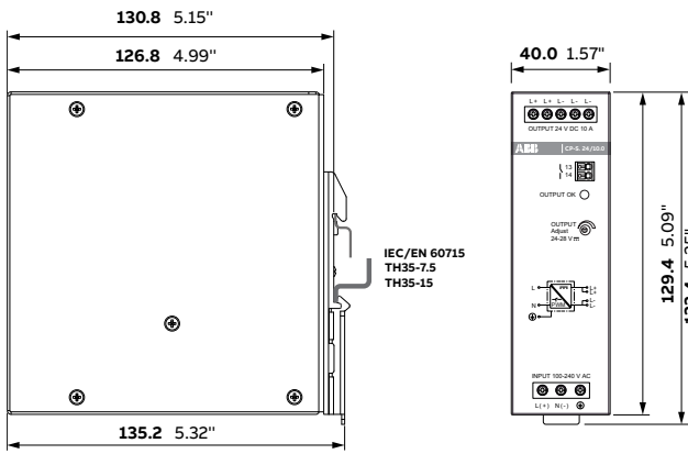
CP-S.124/10.0
