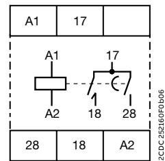
CT-SDD.22
