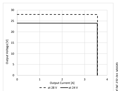
CP-S.1 24/3.0
