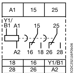
CT-AHD.22
