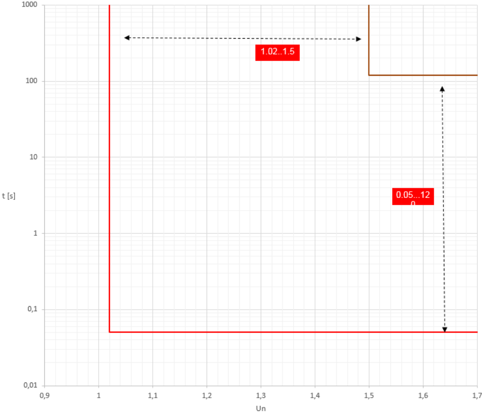
OV 曲线 OV2 曲线
