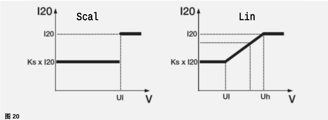
图 20 有关检查与模拟各参数脱扣时间的说明，请参阅：
