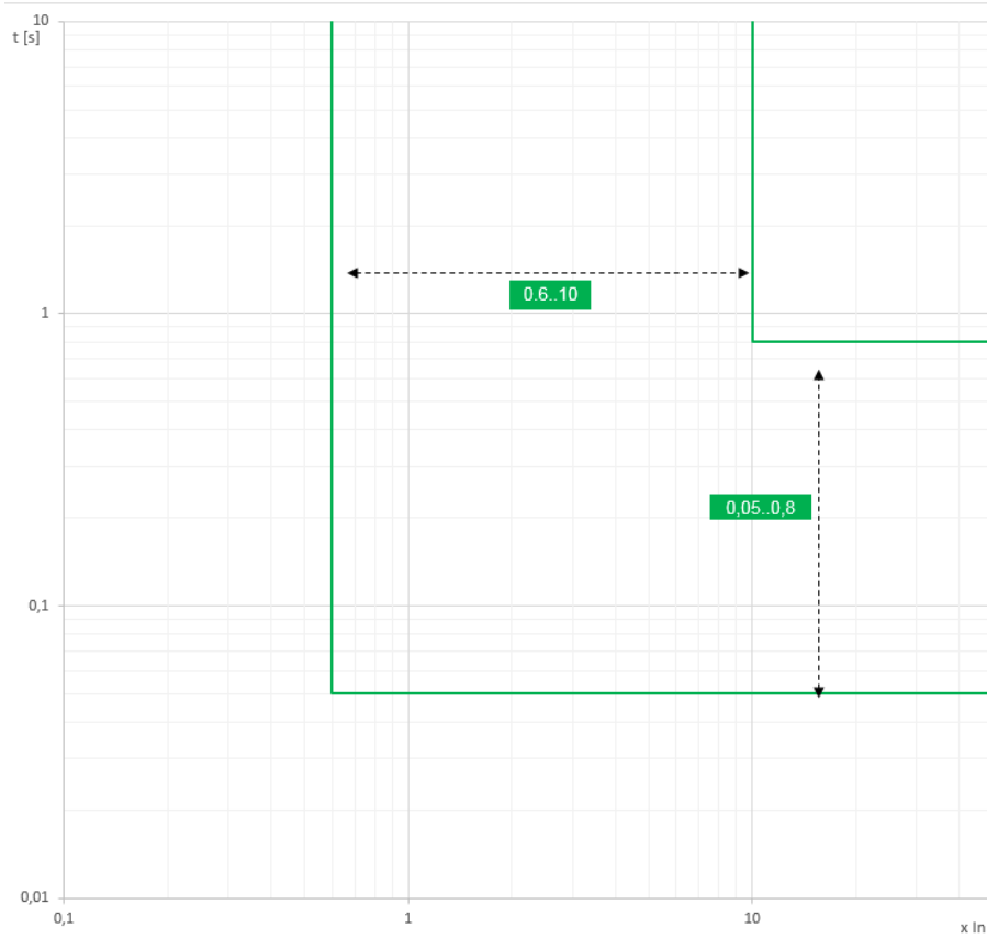
S 曲线 (t= k) 曲线 S2
