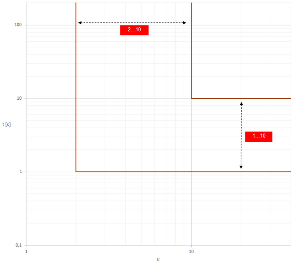
R JAM 曲线 R STALL
