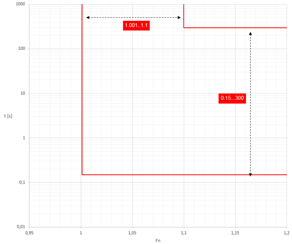
OF 曲线 OF2 曲线
