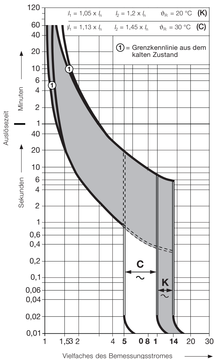
Abb. 5 Auslösekennlinien C/K im Vergleich
