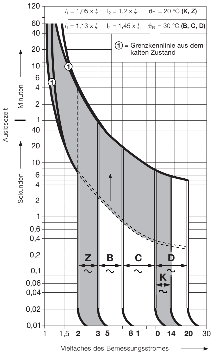
Abb. 3 Auslösecharakteristiken im Vergleich
