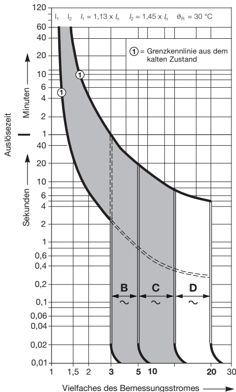
Abb. 7 Auslösekennlinien B/C/D/K/Z im Vergleich
