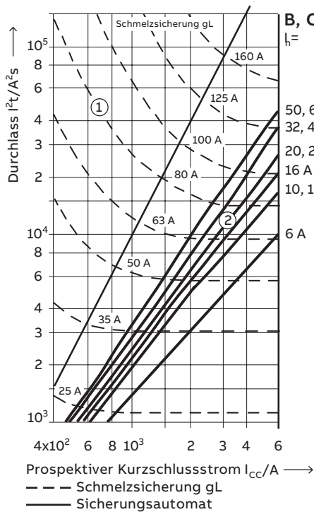
Abb. 1 Durchlassenergie I^2t
