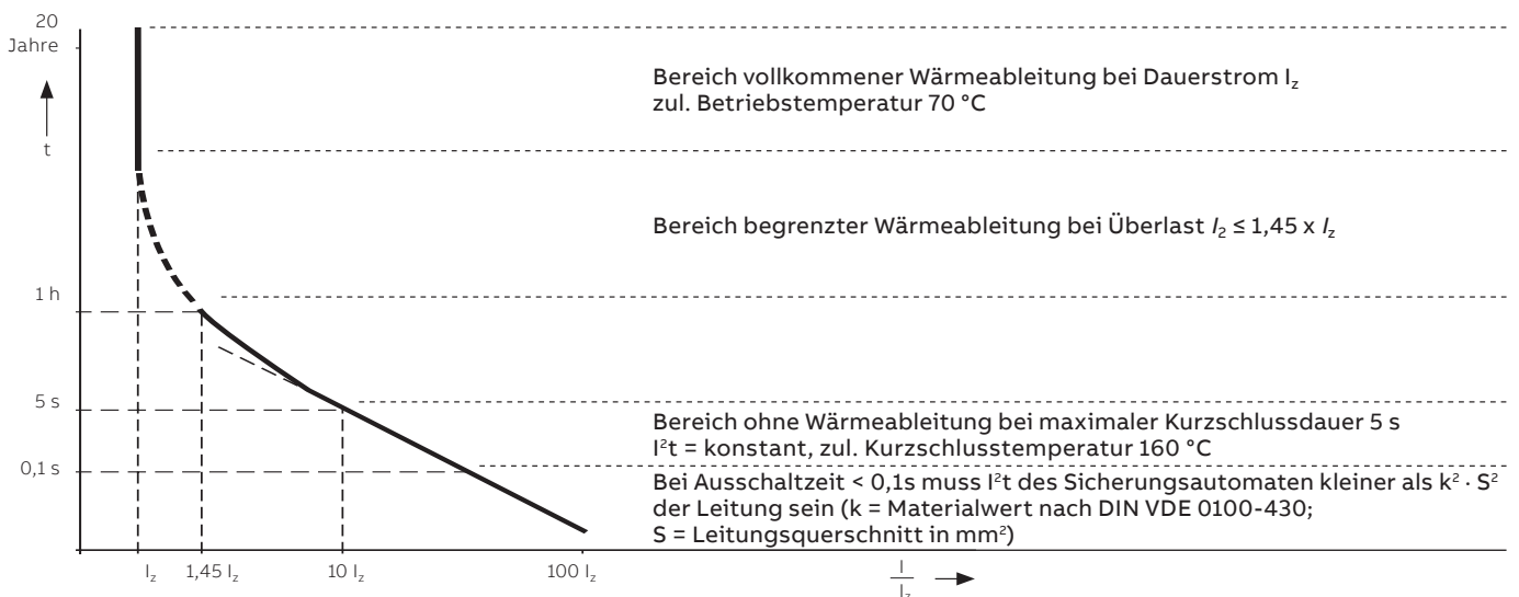
Abb. 2 Grenzbelastungskennlinie für PVC-isolierte Leitungen
