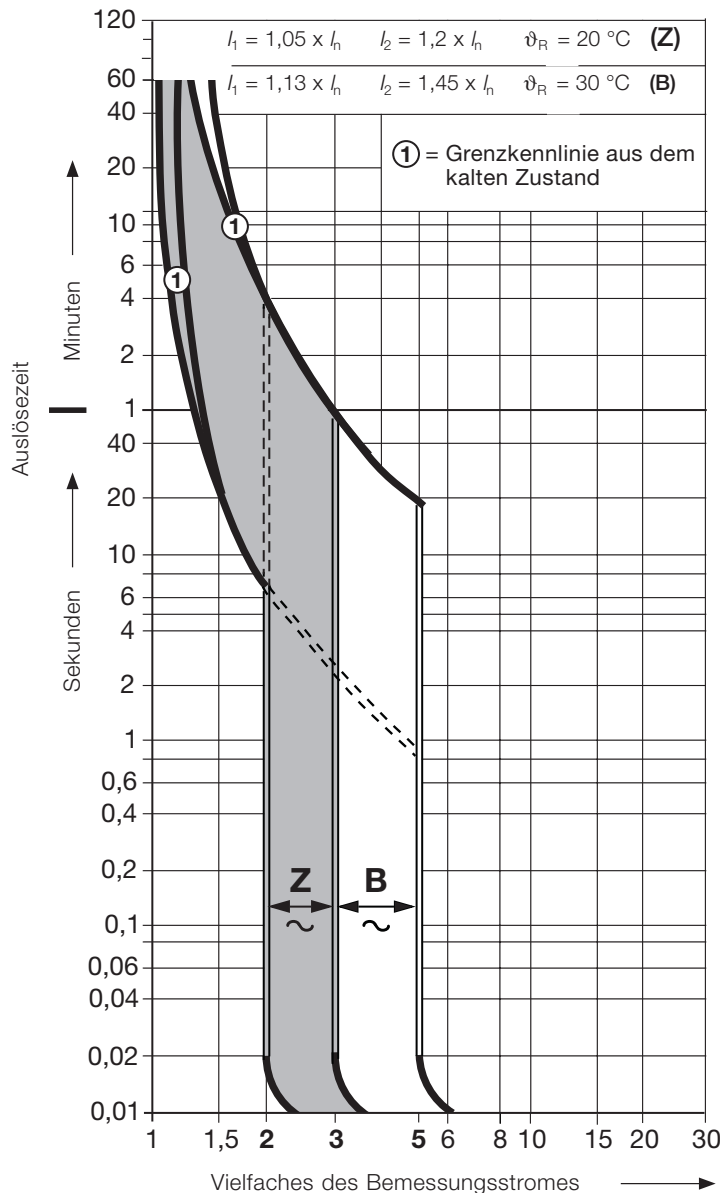
Abb. 4 Auslösekennlinien B/Z im Vergleich
