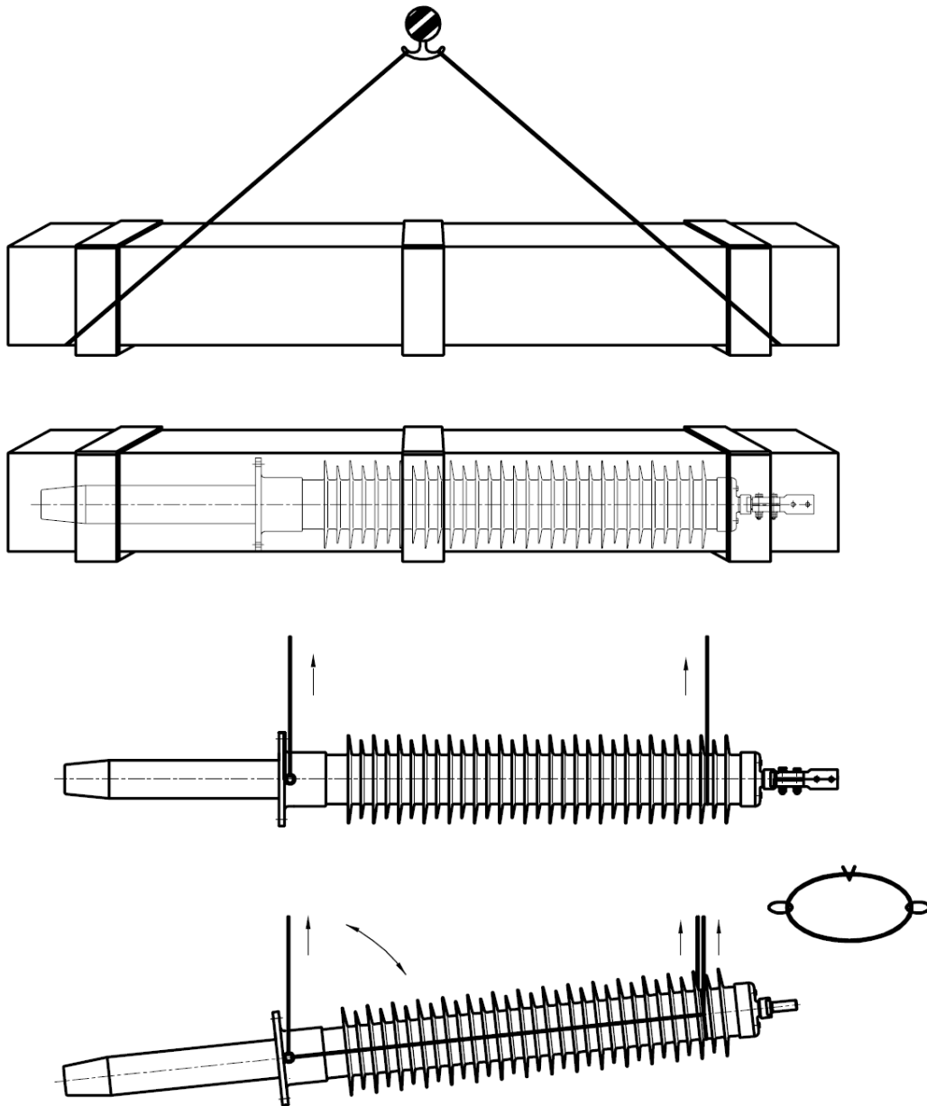
Рис. 2 Подъем ввода
