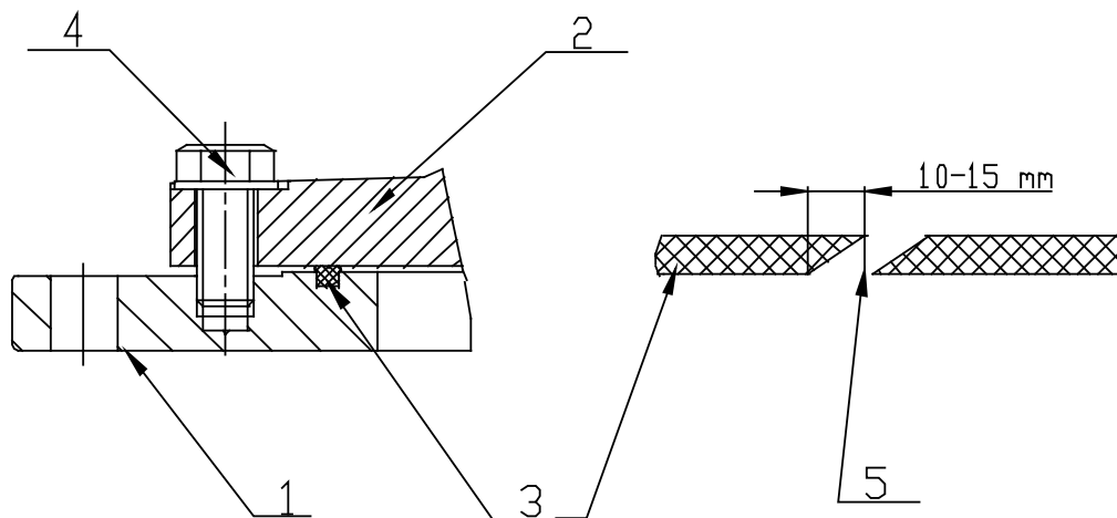
Рис. 3 Монтаж переходного фланца
