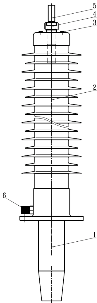
Рис. 1 Конструкция ввода
