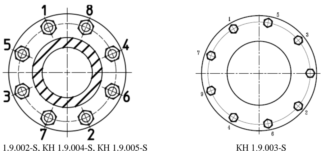
Рис. 6 Порядок крепления фланца
