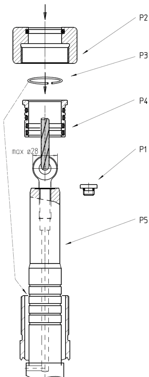
Рис. 4 Установка ввода на трансформатор
