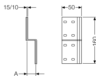
Raccordo di riduzione sinistro
