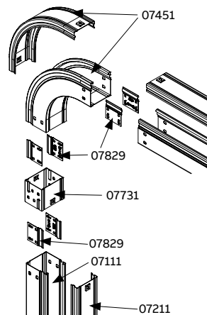
Curva esterna a 90°
