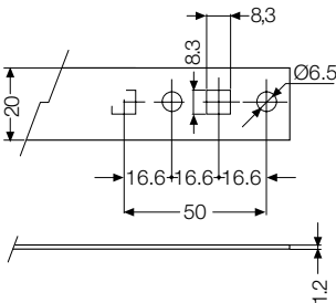
Bandelle forate leggere
