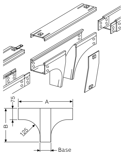
Derivazione a "T" verticale con variazione di piano
