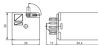
CR-U con 3 contactos
