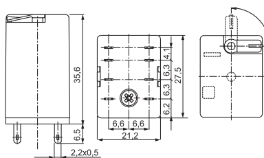
CR-M con 2 contactos
