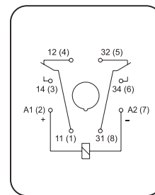
CR-U con 2 contactos
