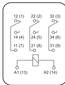
CR-M con 3 contactos
