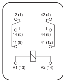
CR-M con 2 contactos
