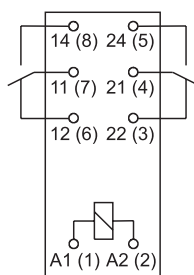
CR-P con 2 contactos
