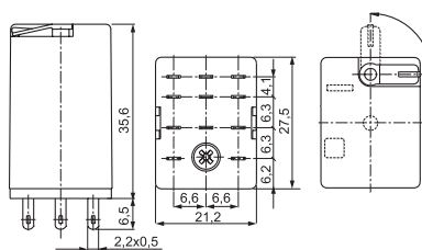
CR-M con 3 contactos
