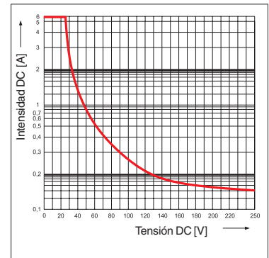
CR-M con 4 contactos
