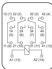
CR-M con 4 contactos
