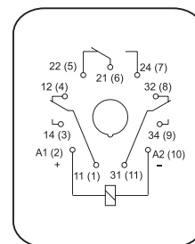
CR-U con 3 contactos
