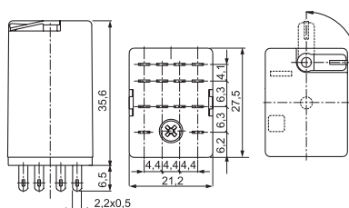
CR-M con 4 contactos
