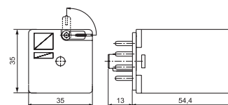
CR-U con 2 contactos
