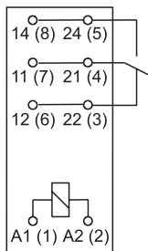
CR-P con 1 contacto
