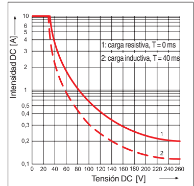
CR-U con 2 y 3 contactos
