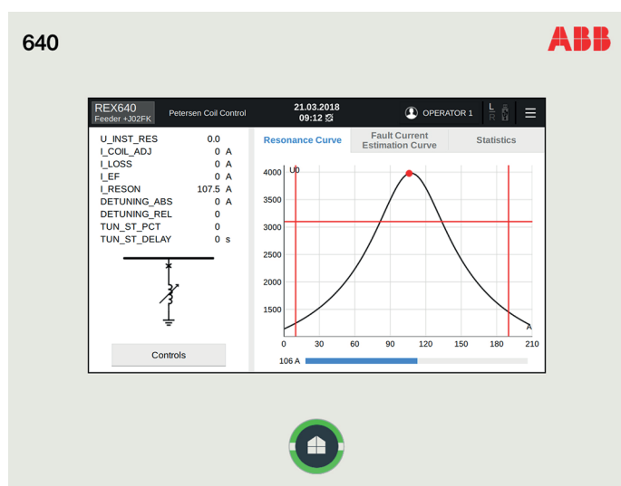
Figure 16. Page de contrôle des bobines Petersen
