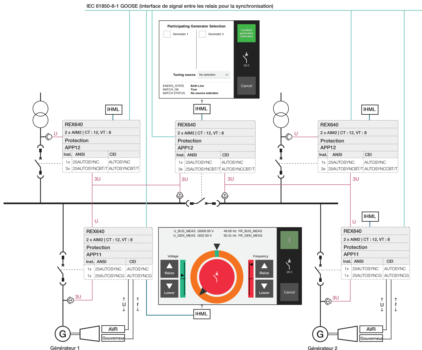
Figure 10. Application d'autosynchroniseur
