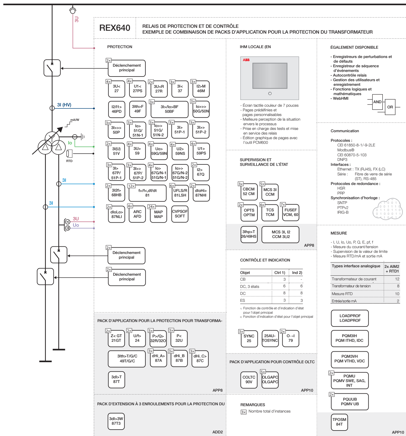
Figure 8. Application de transformateur
