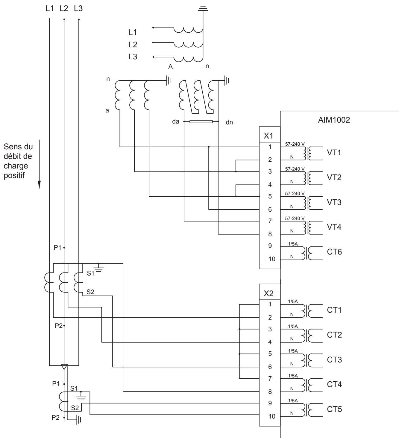
Figure 23. Module AIM1002
