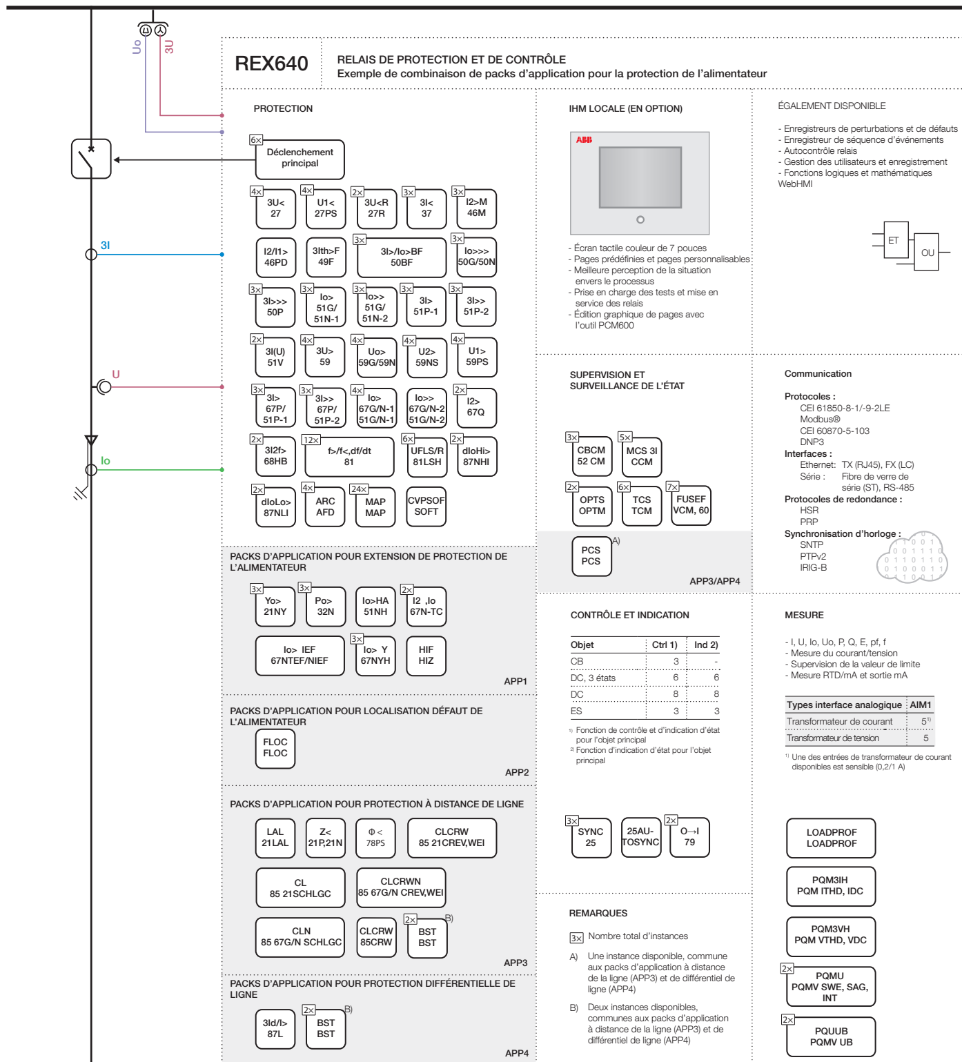
Figure 7. Application des départs et des arrivées
