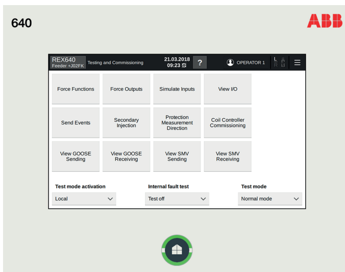
Figure 4. Support de test et de mise en service dans l'IHML locale
