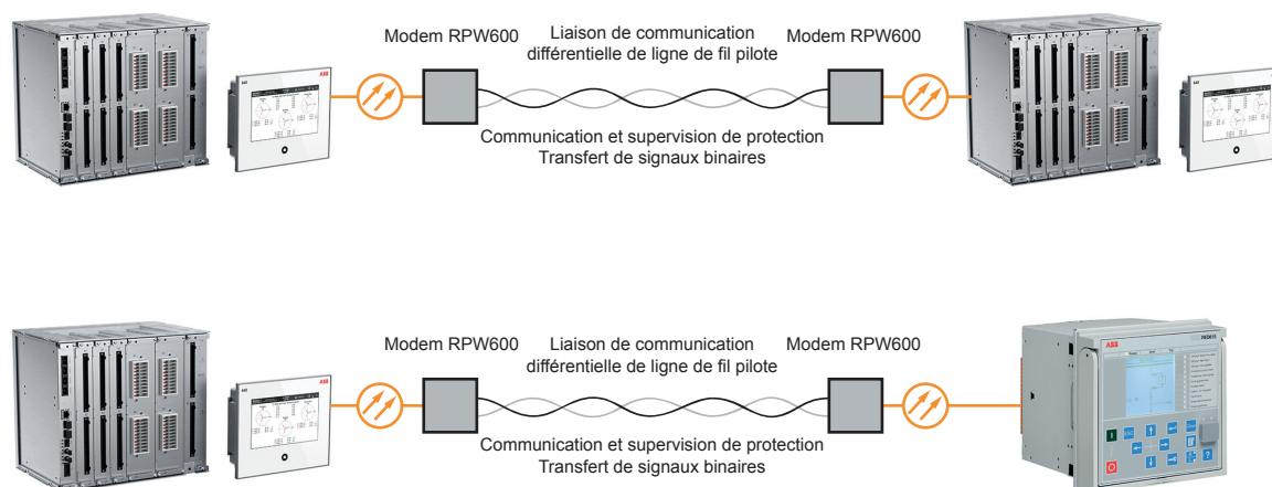
Figure 21. Liaison de communication de protection par fil pilote
