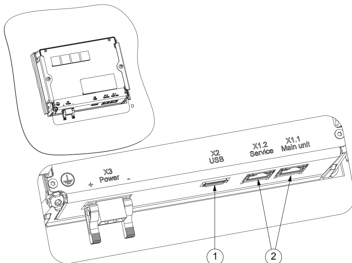
Figure 6. Connecteurs IHML
