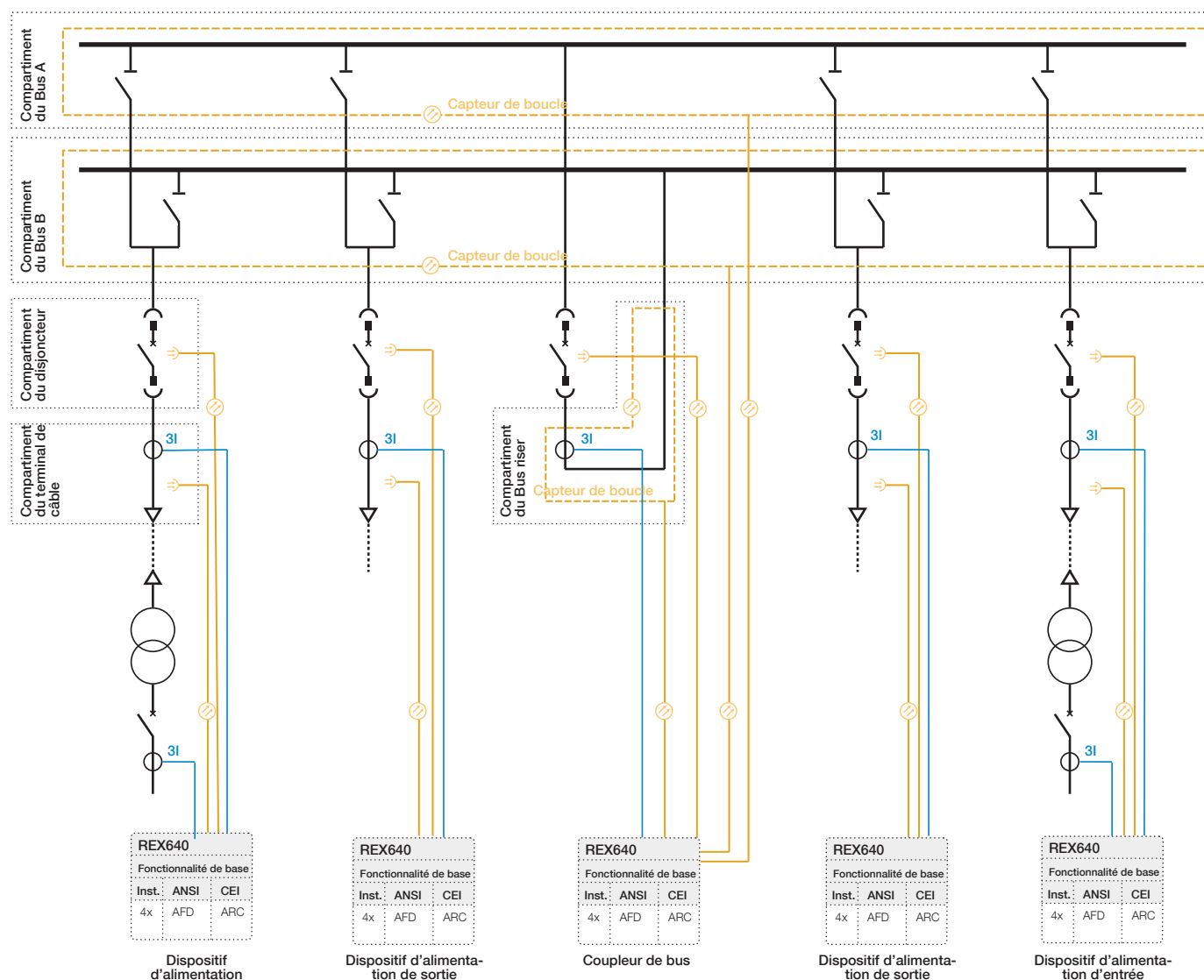
Figure 12. Application de protection contre les coups d'arc
