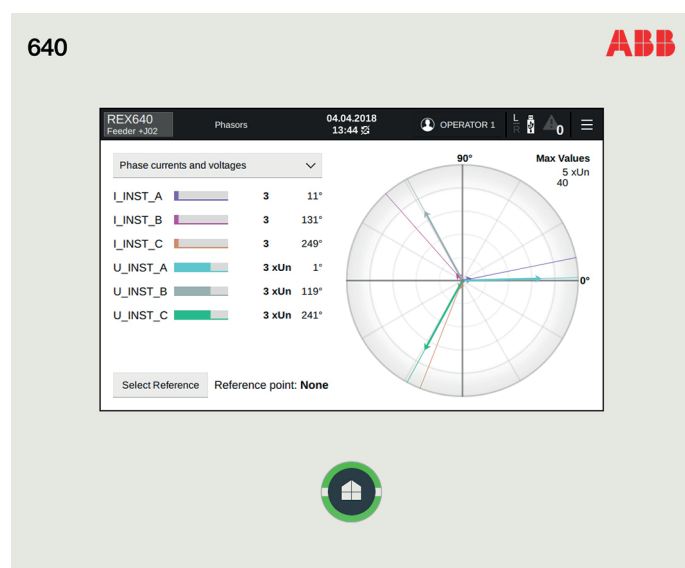
Figure 3. Présentation de phase des mesures comme exemple des pages de l'IHML locale
