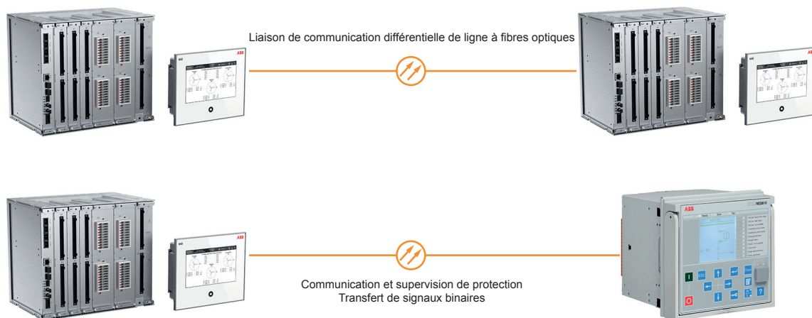
Figure 20. Liaison de communication par fibre optique
