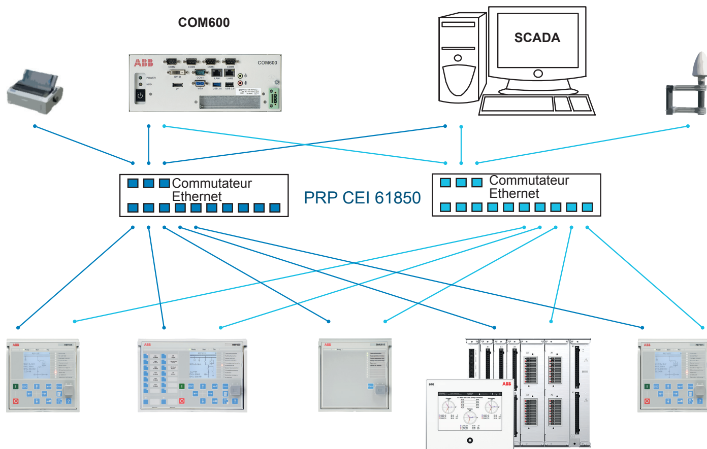
Figure 18. Solution du protocole de redondance parallèle (PRP)
