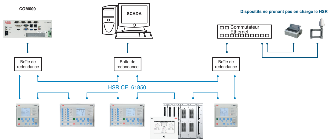
Figure 19. Solution de redondance transparente de haute disponibilité (HSR)
