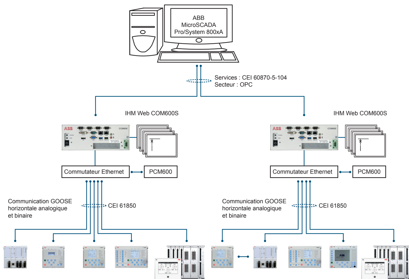
Figure 15. Exemple de réseau de distribution ABB à l'aide de relais Relion, du COM600S et du MicroSCADA Pro/système 800xA
