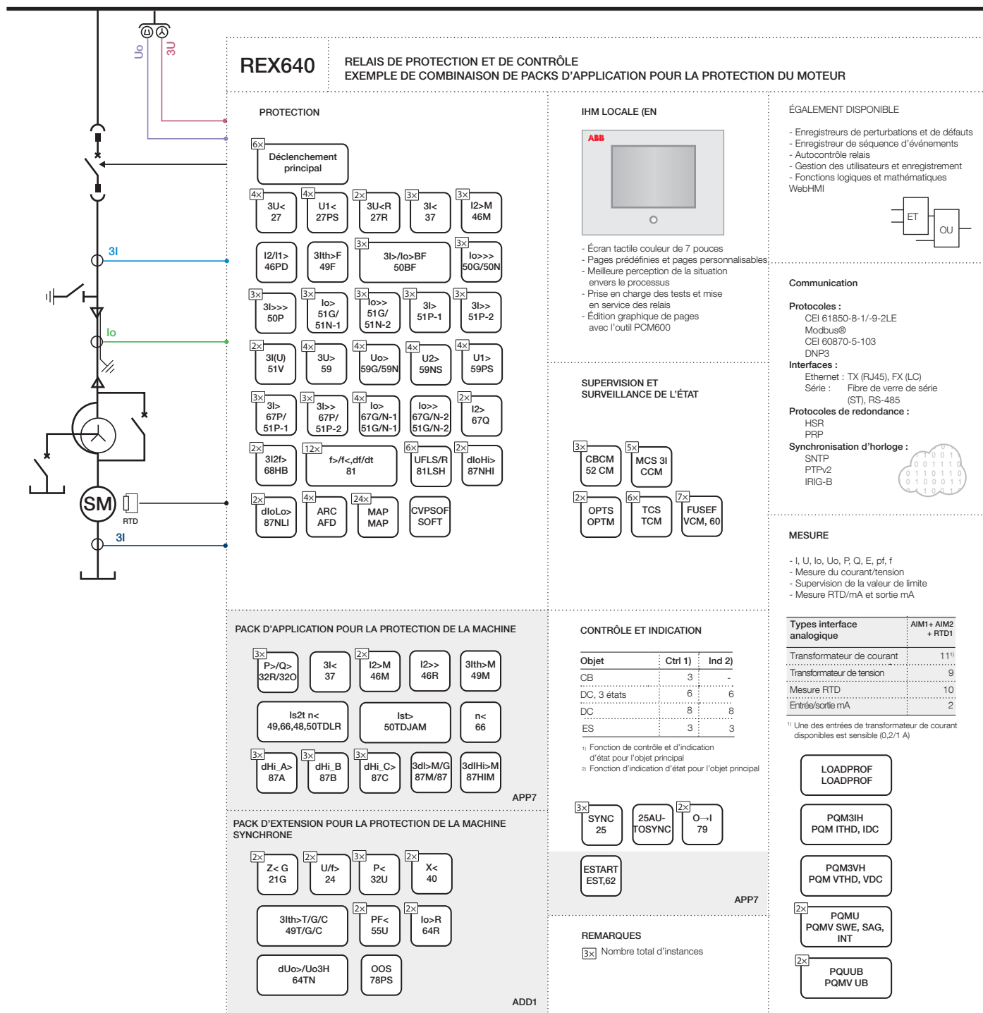
Figure 9. Application de moteur
