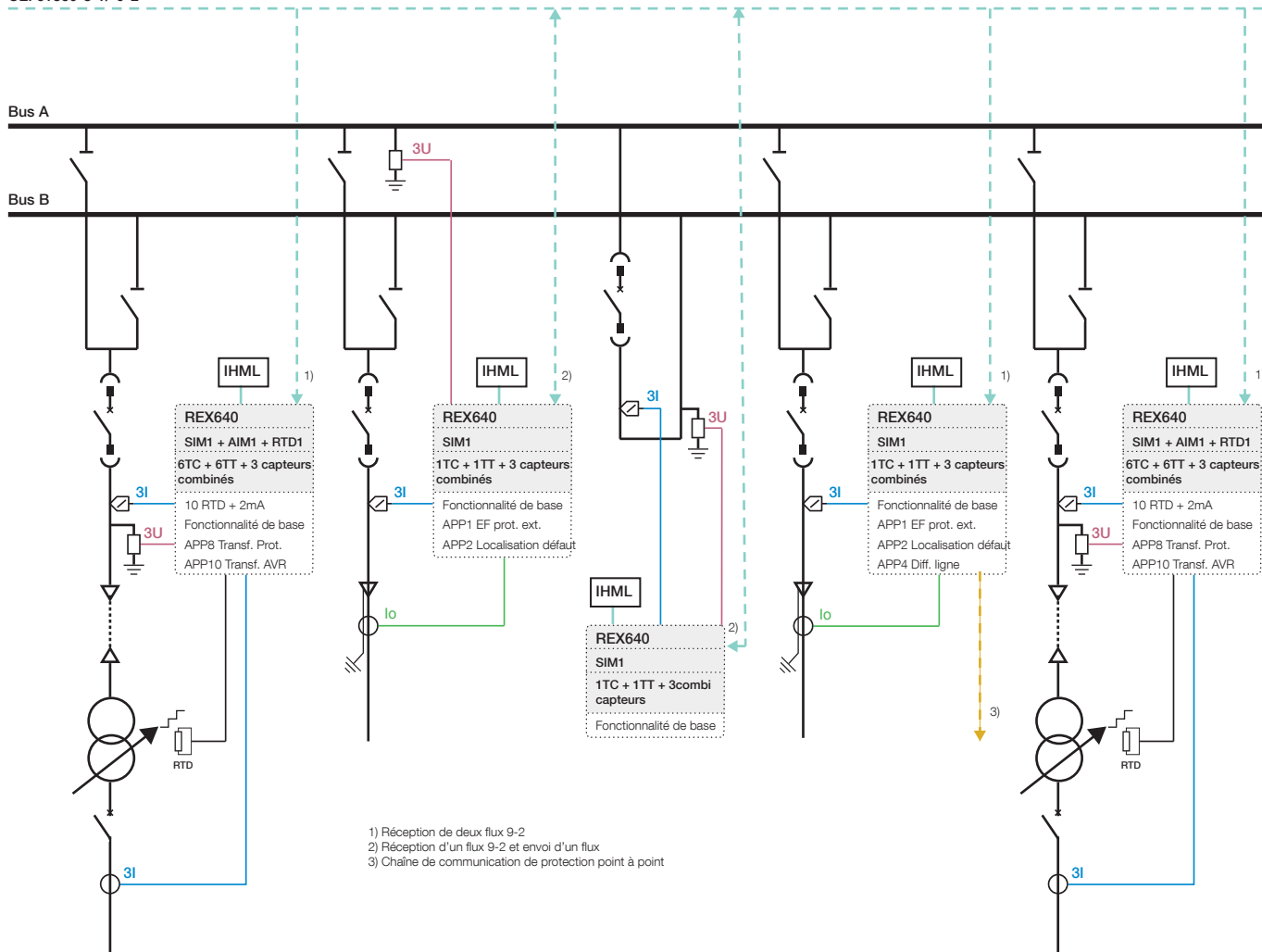
Figure 14. Application d'appareillage de commutation numérique
