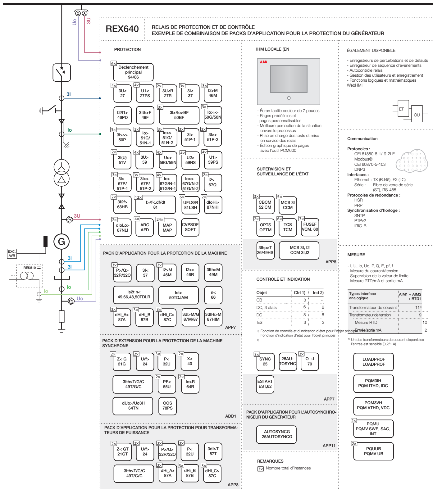
Figure 13. Application de générateur
