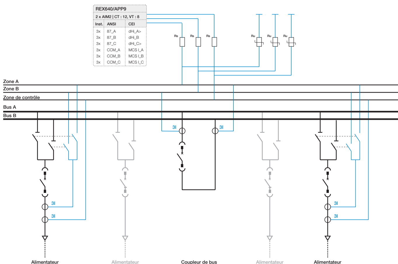
Figure 11. Application de protection de jeux de barres
