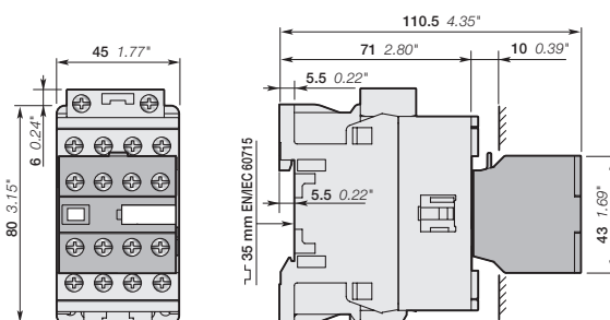
AF16 + CA4 4-poliger Hilfskontaktblock
