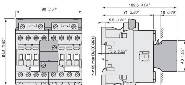
AF16 + VEM4 Mechanischer und elektrischer Verriegelungssatz
