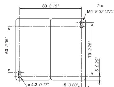
AF16 + VEM4 Mechanischer und elektrischer Verriegelungssatz
