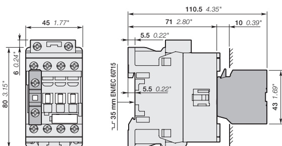
AF16 + CA4, CC4 1-poliger Hilfskontaktblock
