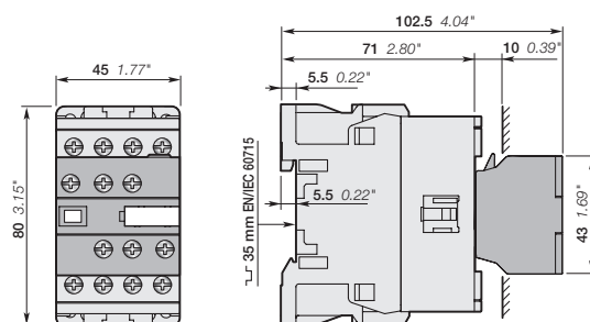
AF16 + CAT4 2-poliger Hilfskontaktblock und Spulenanschlussklemmenblock
