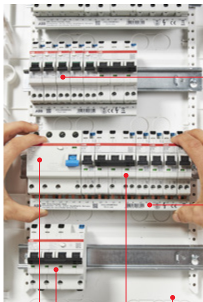
Disjoncteur différentiel FI/LS DSX301C
