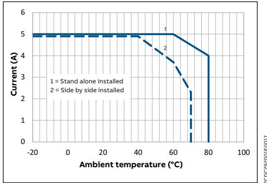
MOS-FET output CR-P
