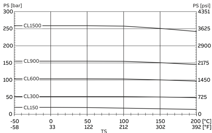
Рисунок 15. Фланец ASME из Nickel-Alloy C4 (2.4610) или Nickel-Alloy C22 (2.4602) до DN 200 (in.)
