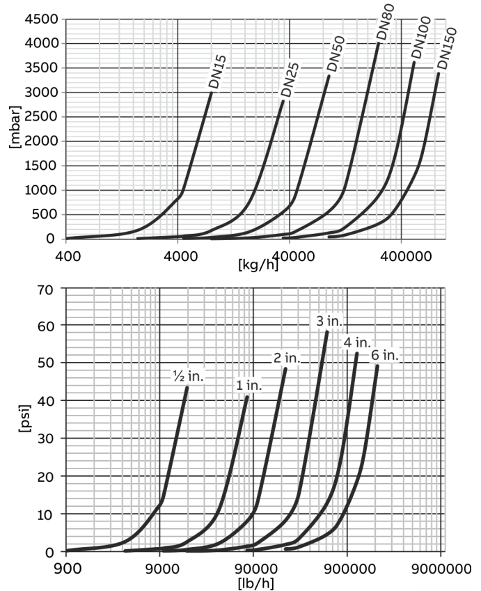
Рисунок 11. Характеристика потери давления (измерена в воде, вязкость: 1 мПа·с)
