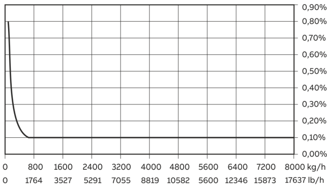
Рисунок 10. Погрешность измерений FCx150 DN 15 (пример)
