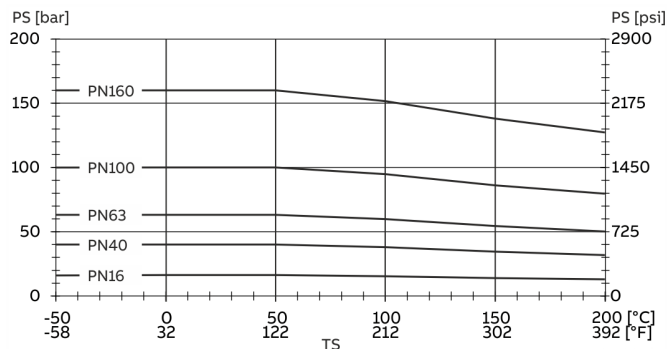
Рисунок 12. Фланец DIN из нержавеющей стали 1.4571 / 1.4404 (316Ti / 316L) до DN 200 (8 in)
