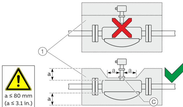
Рисунок 7. Монтаж при T_{medium} от -50^{\circ}\text{C} до 205^{\circ}\text{C} (от -58 до 400^{\circ}\text{F} )
