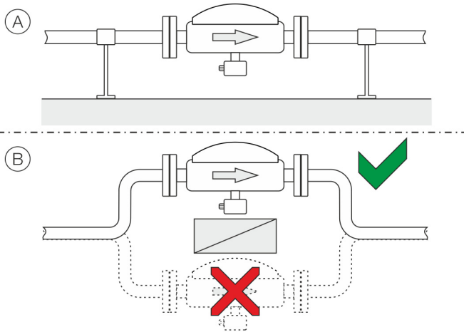
Рисунок 5. Горизонтальный монтаж
