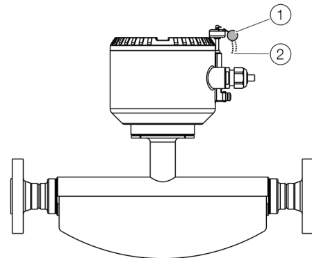
Рисунок 8: Опломбирование согласно MID / OIML R117 (пример)
