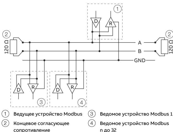
Рисунок 20: Обмен данными по протоколу Modbus
