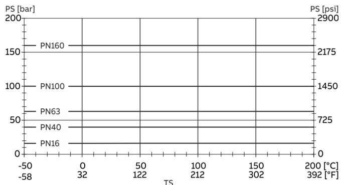
Рисунок 14. Фланец DIN из Nickel-Alloy C4 (2.4610) или Nickel-Alloy C22 (2.4602) до DN 200 (8 in)
