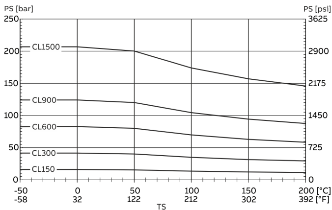
Рисунок 13. Фланец ASME из нержавеющей стали 1.4571 / 1.4404 (316Ti / 316L) до DN 200 (8 in)
