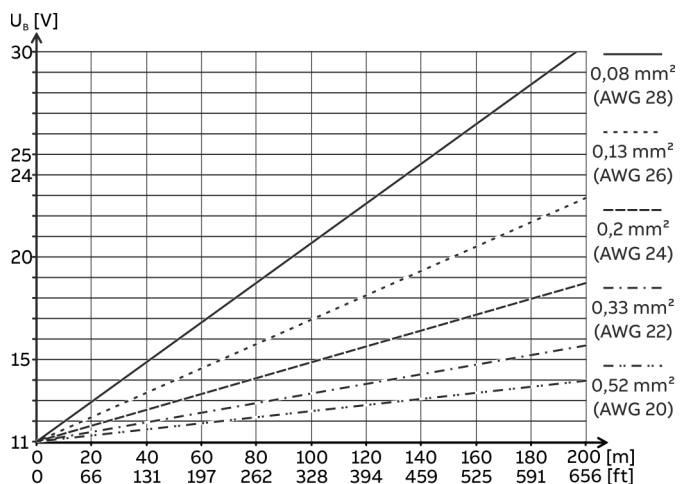
Рисунок 18. Максимальная длина кабеля (примеры)
