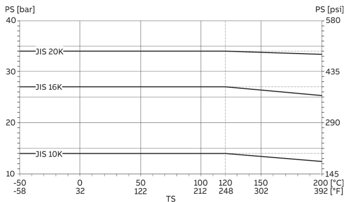
Рисунок 16. Фланец JIS B2220 из нержавеющей стали 1.4435 или 1.4404 (AISI 316L), Nickel-Alloy C4 (2.4610) или Nickel-Alloy C22 (2.4602)
