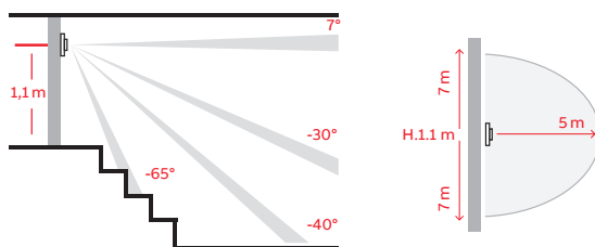
Flex Multi 180° tunnistusalue
