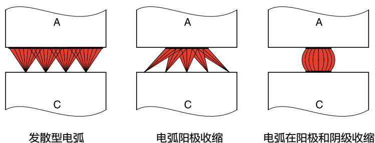
电弧在真空灭弧室中从发散型到收缩型的转化过程的示意图
