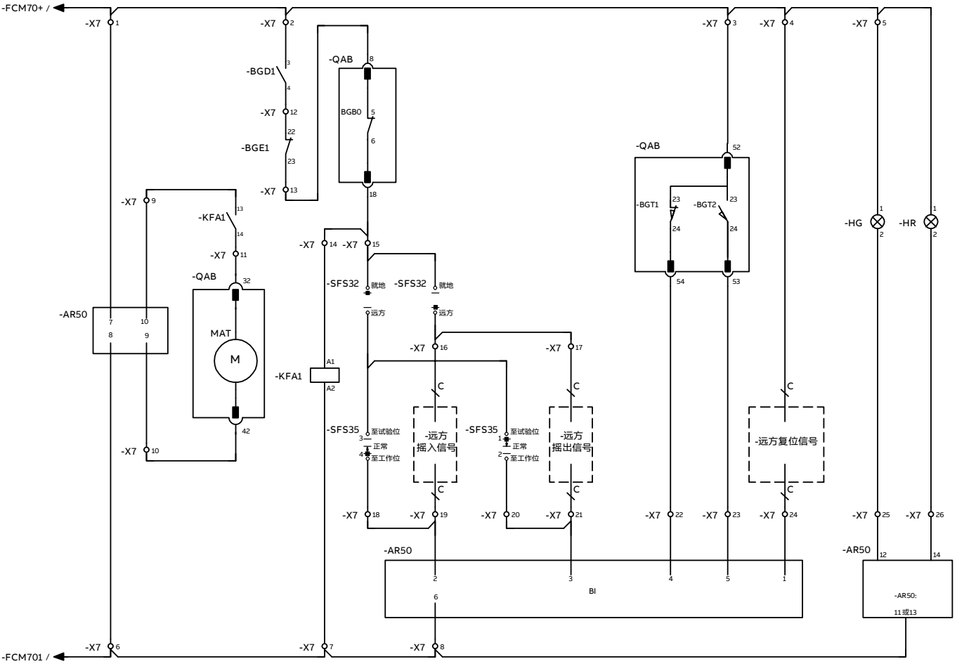
MDC2电机驱动手车数字控制单元工程应用图
