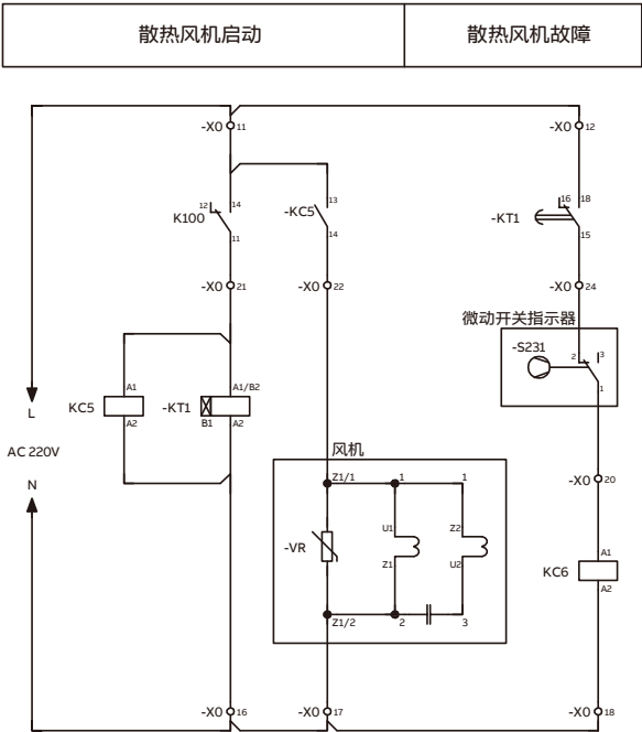
断路器风机使用典型工程应用图
