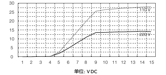
分、合闸脱扣器伏安特性曲线 单位: mA
