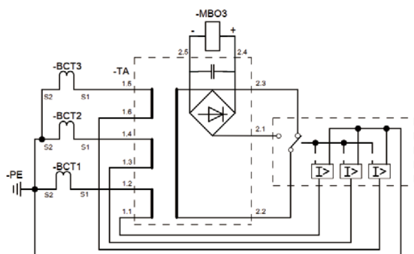
图 1 三相回路
