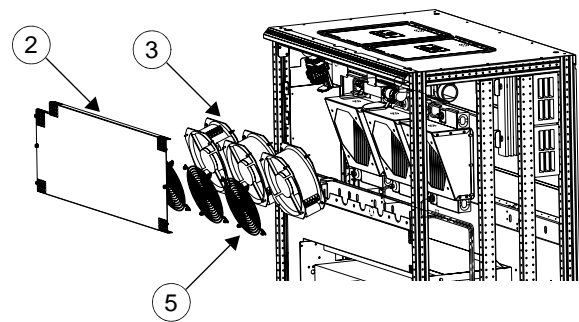
1000 mm 宽机柜
