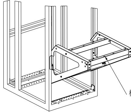
横梁的固定
