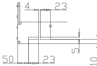
卡槽的间距
