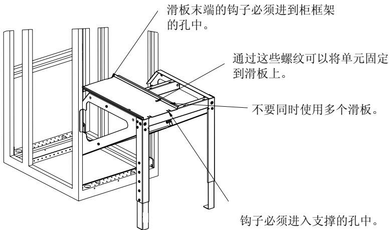
滑板和支脚
