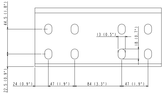
输入母排尺寸 (1000 mm 宽断路器柜体)
