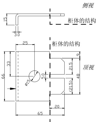
夹具尺寸 (毫米)
