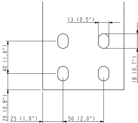
进线端子尺寸 (600 mm 宽断路器柜体)
