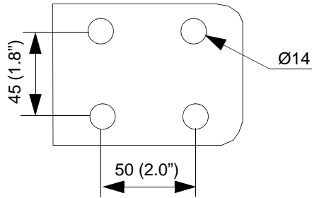
进线端子尺寸 (600 mm 宽断路器柜体)
