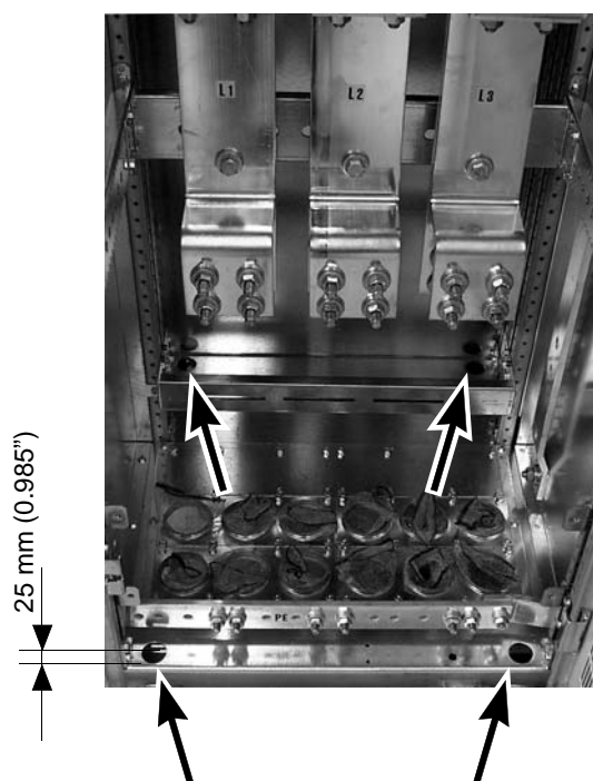
柜内的固定孔 (箭头所示)
