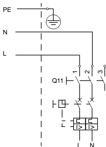
辅助控制电路电源 ( 单元为 UPS 安装可选项 +G307 UPS )
