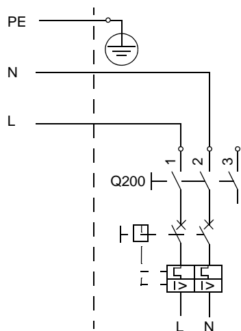
控制电路的供电电源 (单元为 UPS 加可选项 +G307)
