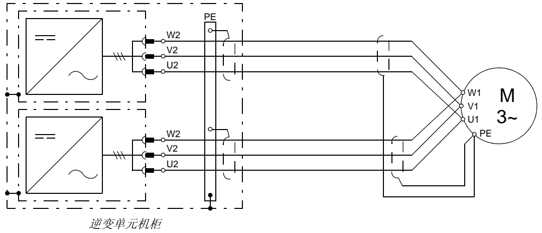
接线图 - 并联逆变模块为驱动一台电机
