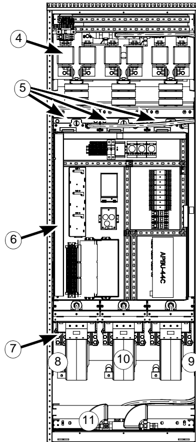
3xR8i, 柜门打开
