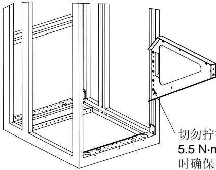
三角支撑的固定
