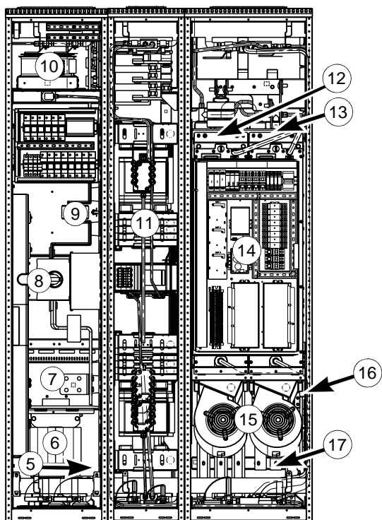
柜门打开
