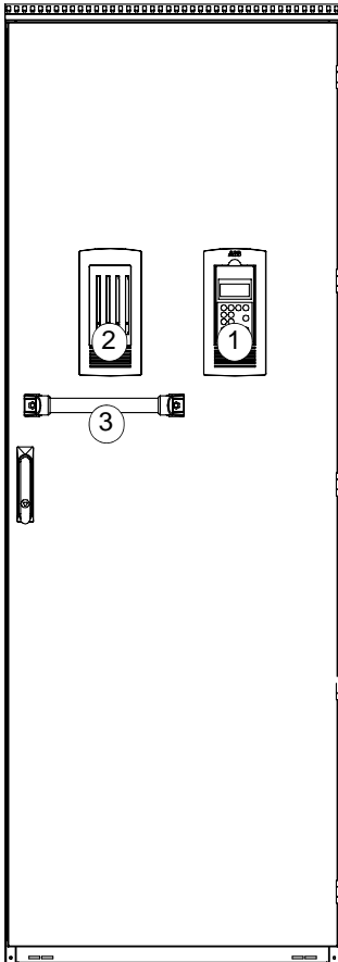
3xR8i, 柜门关闭
