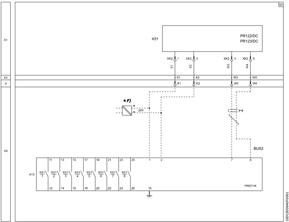
PR021/K信号单元
