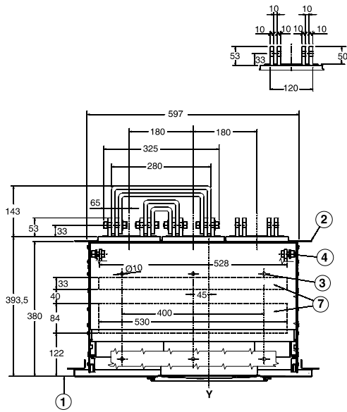
E4 III 视图 A
