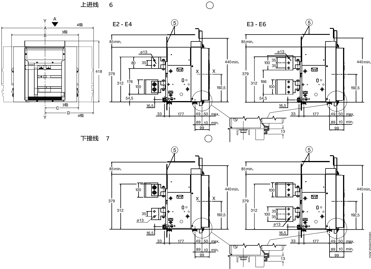
基本型（垂直后接线端子）
