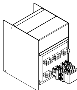
上进线
