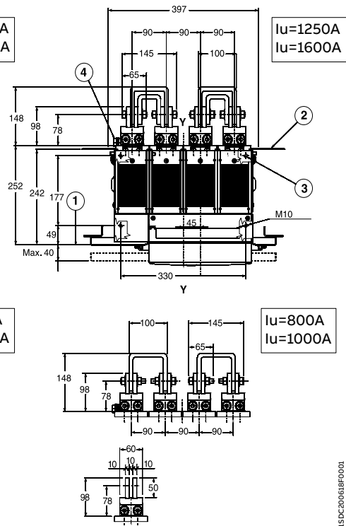
E2 IV 视图 A
