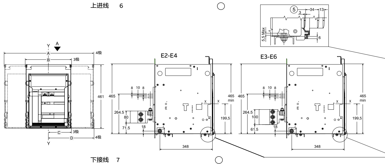
基本型（水平后接线端子）
