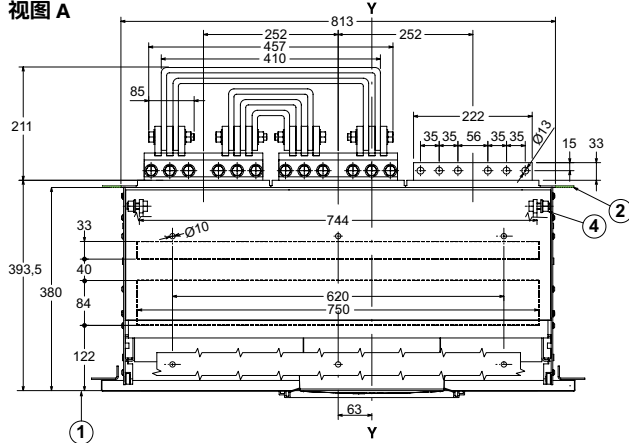
E6 III 视图 A
