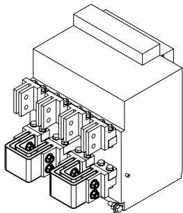
3D后视图
