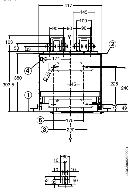
E2 IV 视图 A
