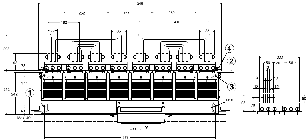
E6 IV 视图 A
