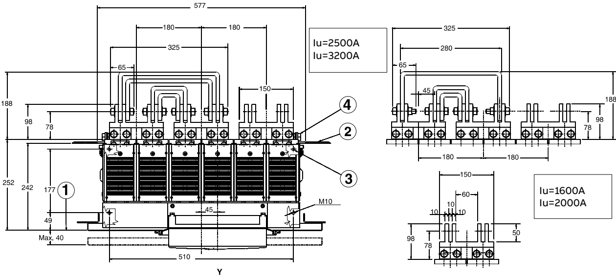
E4 III 视图 A
