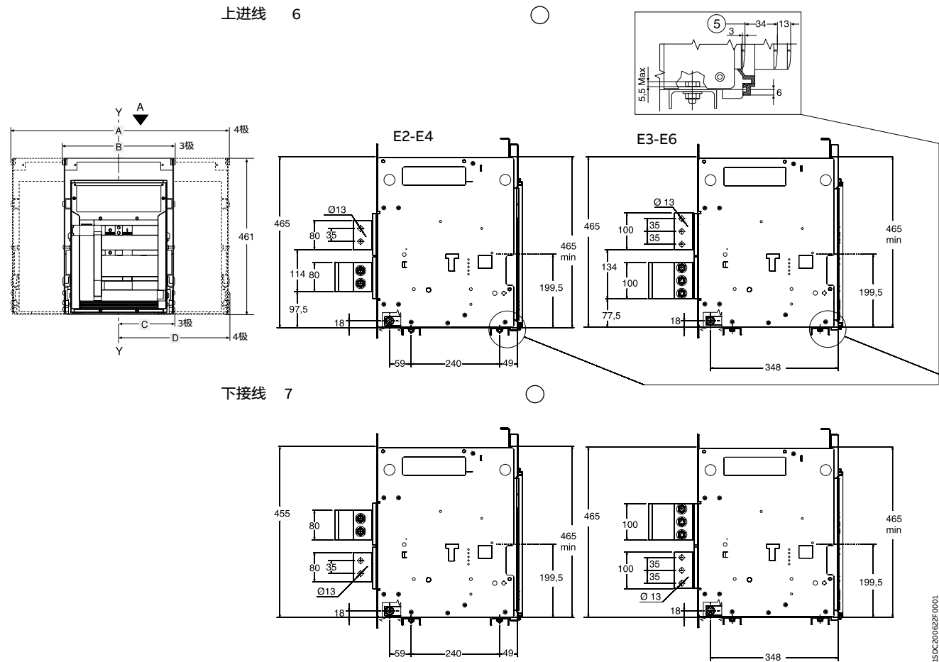
基本型（垂直后接线端子）
