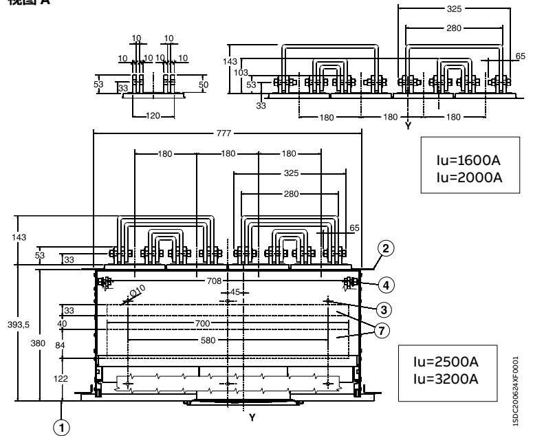
E4 IV 视图 A
