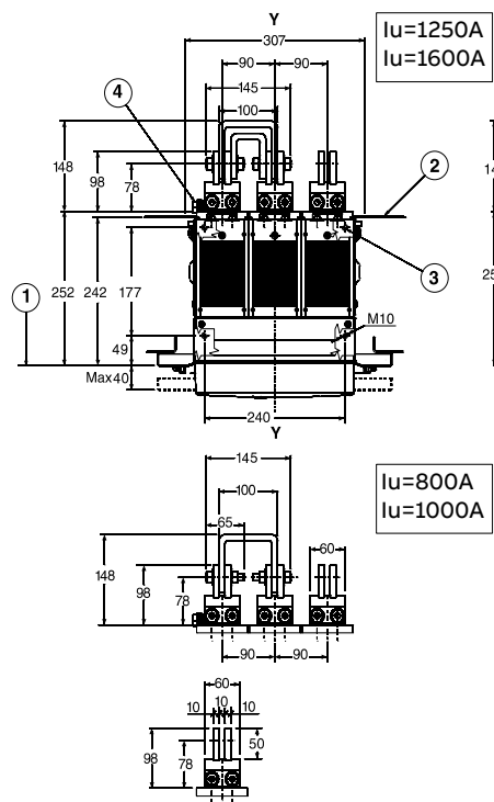
E2 III 视图 A
