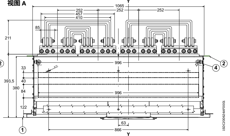
E6 IV 视图 A
