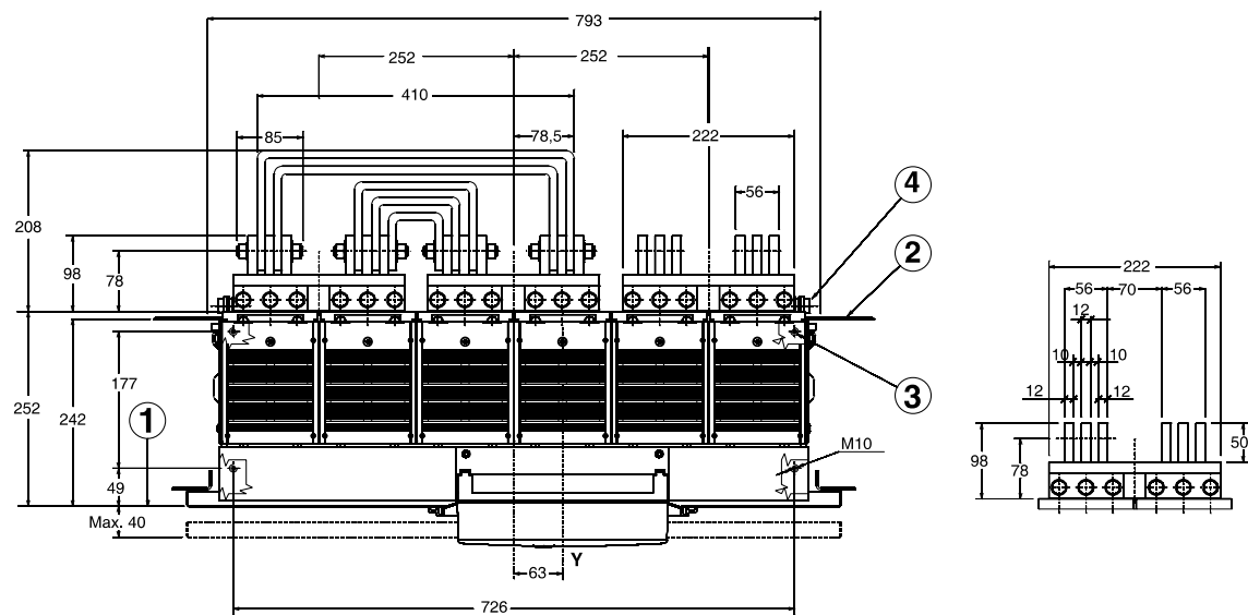
E6 IV 视图 A
