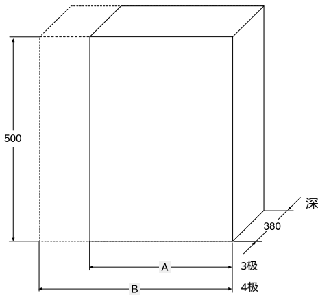
隔室尺寸
