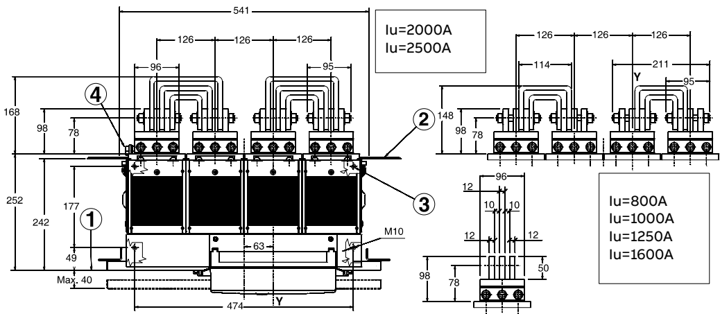
E3 IV 视图 A
