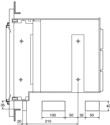
柔性电缆用通孔 (用于机械联锁)
