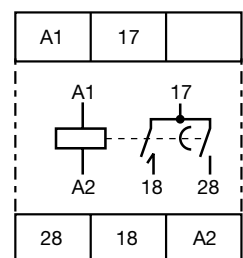
CT-SDD.22
