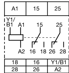
CT-MFD.21
