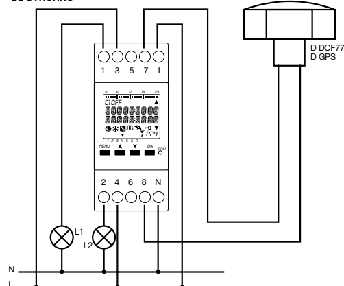
D2 SYNCHRO
