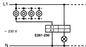
E 261-230
