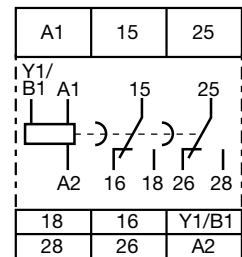
CT-AHD.22
