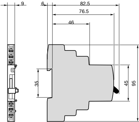
S800-AUX, S800-AUX/ALT
