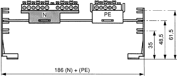
SMO 10
