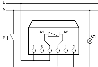
FLR1-12, FLR1-230
