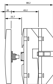
CL-LDC.S..
