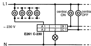
E 261 C-230
