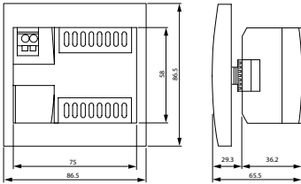
CL-LDC.S..
