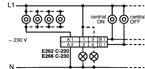
E 266 C-230
