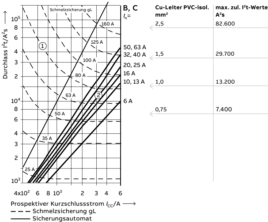
Abb. 2 Durchlassenergie I²t
