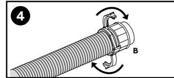
Fermer le mécanisme (B) de verrouillage. Cerrar el mecanismo (B) de bloqueo.
