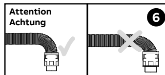
If bending the conduit, please adhere to the recommended bending radius. Beim Biegen des Rohres die vorgeschriebenen Biegeradien einhalten.
