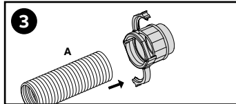
Pousser la gaine (A) à l'intérieur du raccord jusqu'à l'arrêt. Empujar el tubo (A) hasta el final.
