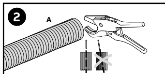
Cut the conduit straight in the corrugation (A). Rohr (A) im Wellental gerade abscheiden.
