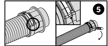
Pour rouvrir, utiliser un tournevis. Utilizar un destornillador para abrir.
