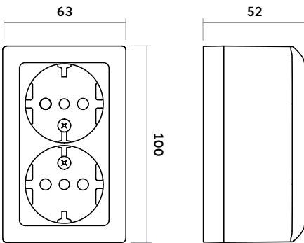
Steckdose 2-fach
