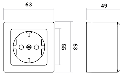
Steckdose 1-fach
