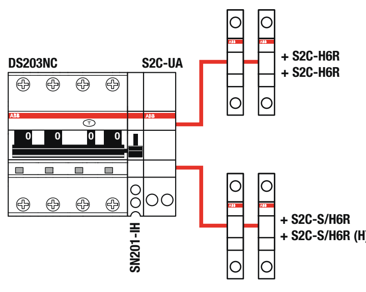
S2C-UA
