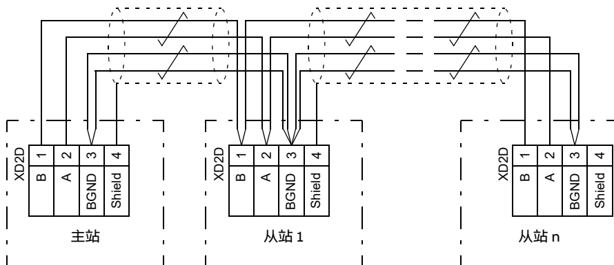
主 / 从电缆接线方式
