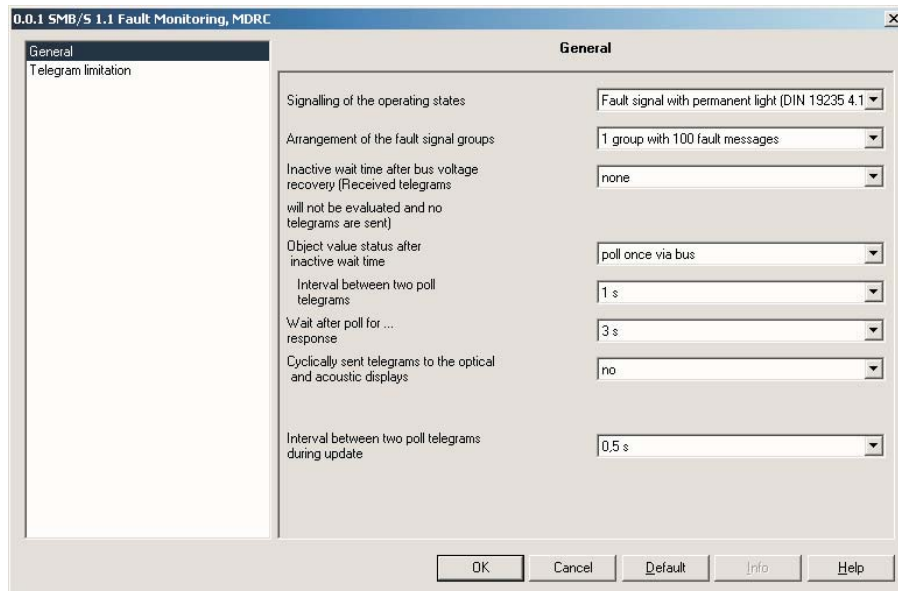
Fig. 4: Parameter window "General"
