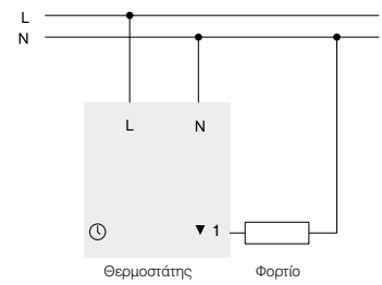
Θερμοστάτης χώρου
