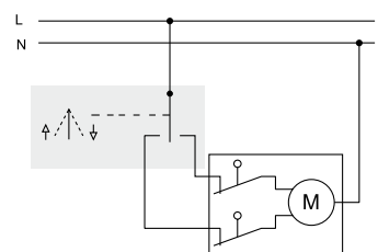
Διακόπτης και μπουτόν ρολών περιστροφικός
