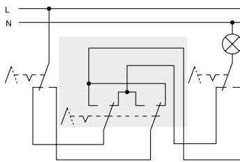
Διακόπτης ενδιάμεσος αλέ-ρετούρ
