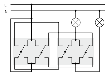
Διακόπτης διπλός αλέ-ρετούρ
