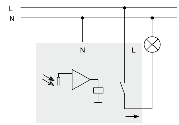
Επιτηρητής παρουσίας ανθρώπων
