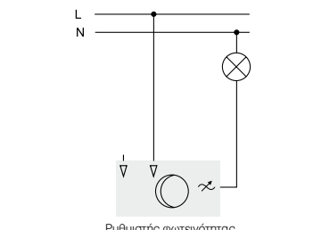
Ρυθμιστής φωτεινότητας (Ροοστάτης)
