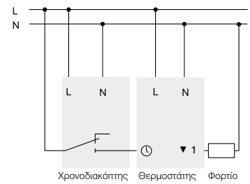
Θερμοστάτης χώρου με χρονοδιακόπτη
