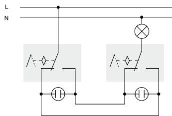
Διακόπτης αλέ-ρετούρ
