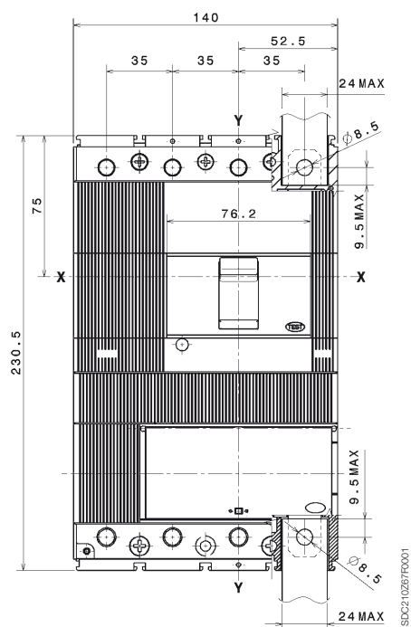
Prises avant avec bloc différentiel
