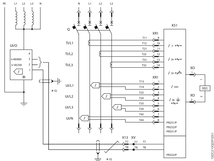
Disjoncteur tétrapolaire avec déclencheur électronique PR231/P, PR232/P, PR331/P ou PR332/P
