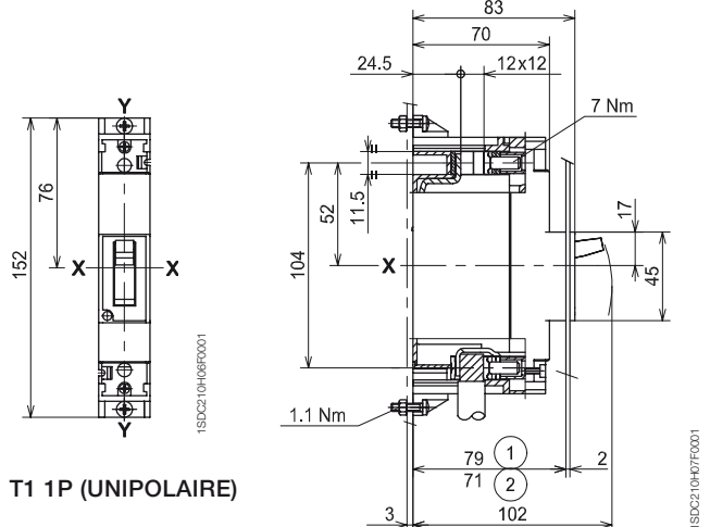
Disjoncteur avec blocs
