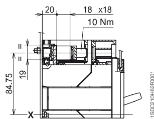
Avant pour câbles en cuivre - FC Cu
