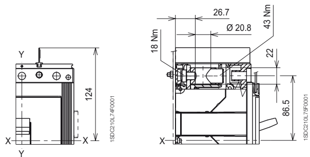
Avant pour câbles en cuivre/aluminium - FC CuAl 2x240 mm 2
