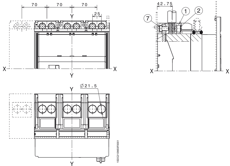
Avant pour câbles en cuivre/aluminium - FC CuAl 4x240 mm 2
