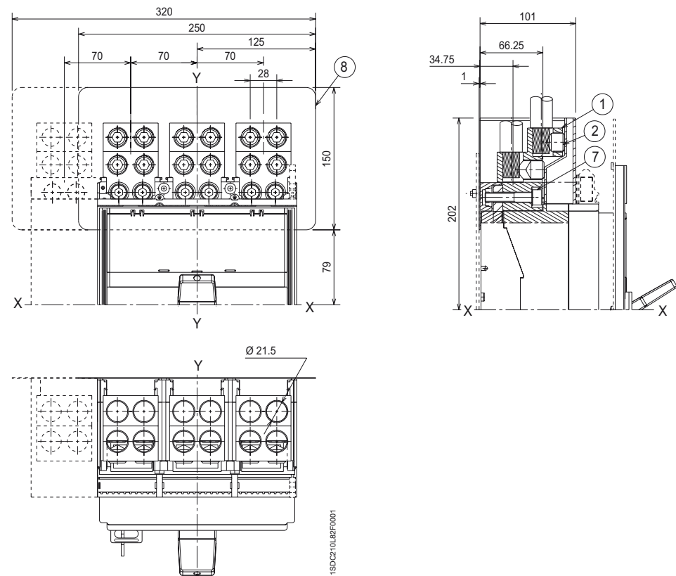
Avant pour câbles en cuivre/aluminium - FC CuAl 4x240 mm 2
