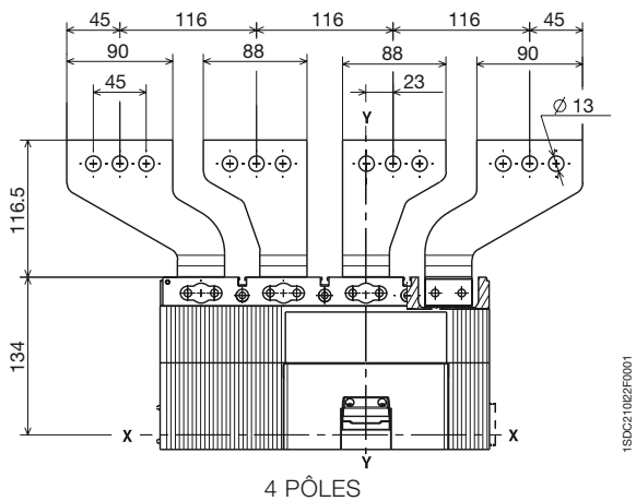
Avant prolongées épanouies - ES
