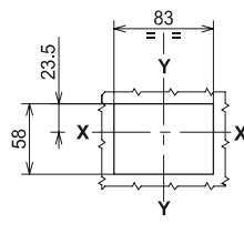
Avec garniture et disjoncteur affleurant (3-4 PÔLES)
