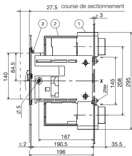
Fixation sur platine
