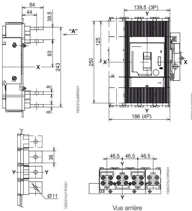
Arrière en barre plate horizontales 630 A - HR
