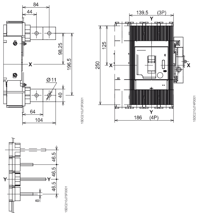
Arrière en barre plate verticales 630 A - VR
