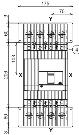
Avant pour câbles en cuivre/aluminium - FC CuAl 240 mm 2
