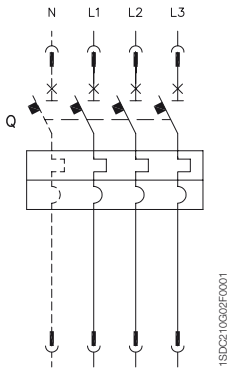
Disjoncteur tripolaire ou tétrapolaire avec déclencheur magnétothermique
