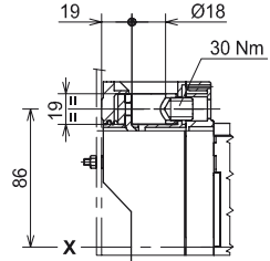
Avant pour câbles en cuivre/aluminium - FC CuAl 185 mm 2
