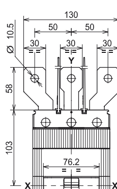
Avant prolongées épanouies - ES
