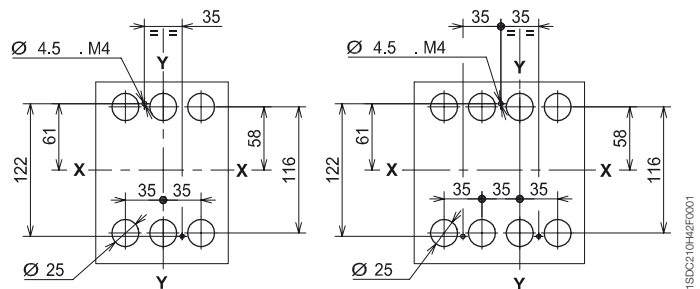
Pour prises arrière
