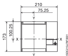
Garniture de porte
