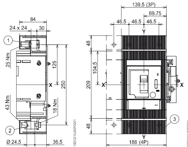
Avant pour câbles en cuivre - FC Cu ou pour câbles cuivre/aluminium - FC CuAl 400 A
