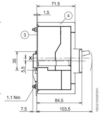
Fixation sur rail DIN EN 50022
