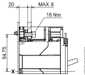
Avant pour câbles en cuivre/aluminium - FC CuAl
