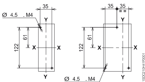
Pour prises avant
