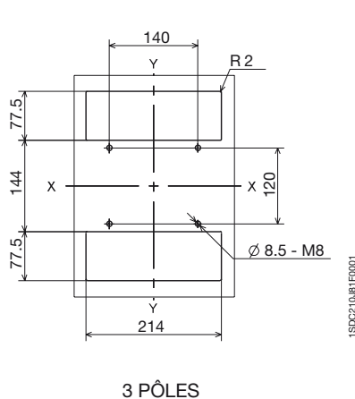
Gabris de perçage de la platine de fixation
