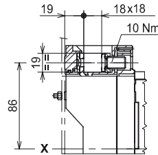
Avant pour câbles en cuivre/aluminium - FC CuAl 240 mm 2
