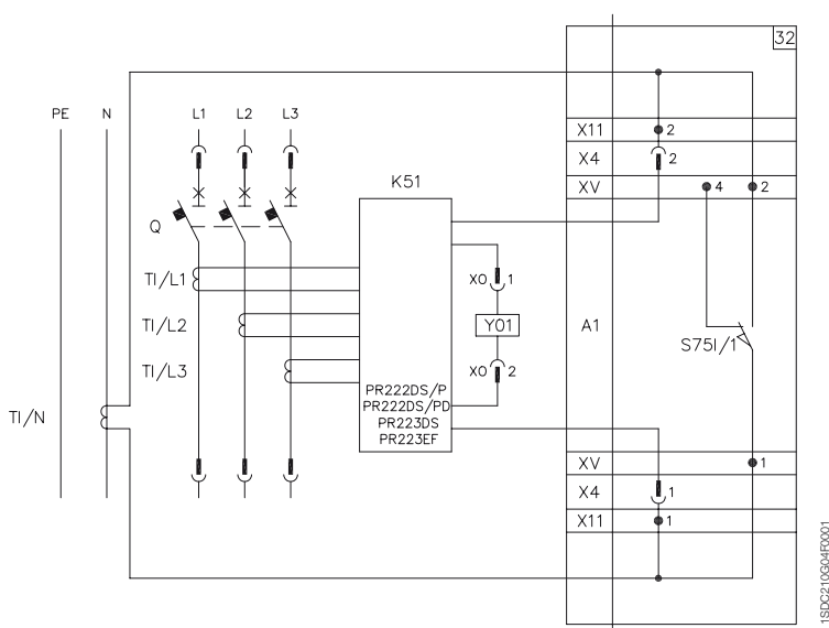
Disjoncteur tripolaire en version débrochable ou débrochable sur chariot avec transformateur de courant sur conducteur neutre extérieur au disjoncteur (pour T4, T5 et T6)
