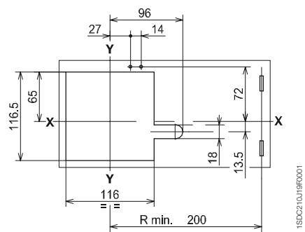
Découpe de face avant
