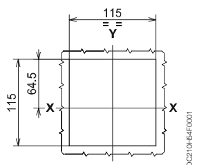
3-4 PÔLES Avec garniture
