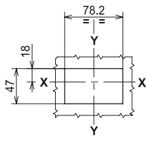
Sans garniture et disjoncteur affleurant (3-4 PÔLES)
