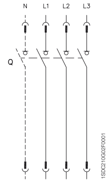
Interrupteur-sectionneur tripolaire ou tétrapolaire)
