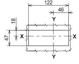
Sans garniture et disjoncteur en saillie (4 PÔLES)
