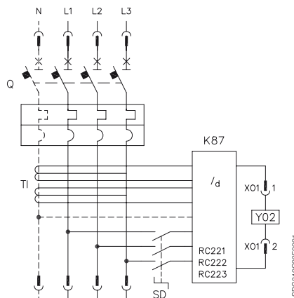
Disjoncteur tripolaire ou tétrapolaire avec bloc différentiel RC221, RC222 ou RC223
