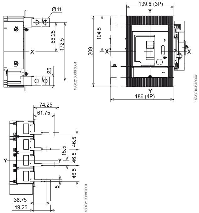
Arrière en barre plate verticales 400 A - VR
