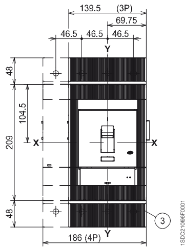
Avant pour câbles en cuivre - FC Cu ou pour câbles cuivre/aluminium - FC CuAl
