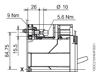
Avant pour câbles en cuivre/aluminium - FC CuAl
