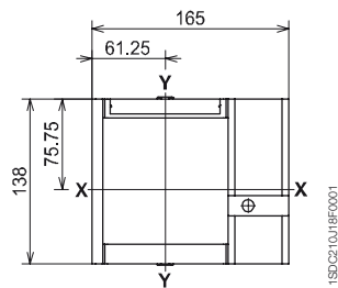
Garniture de porte
