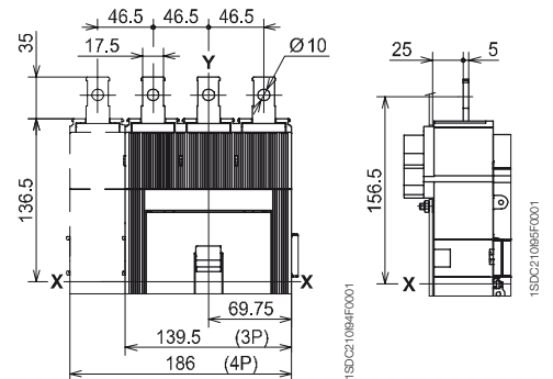
Avant prolongées 630 A - EF
