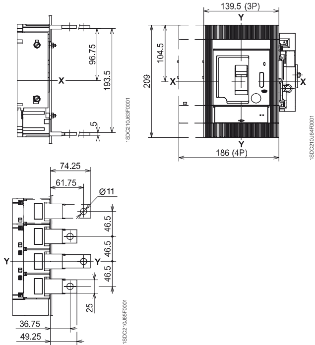
Arrière en barre plate horizontales 400 A - HR
