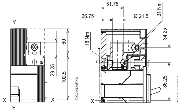
Avant pour câbles en cuivre - FC Cu 2x240 mm 2
