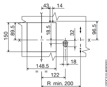
Découpe de face avant
