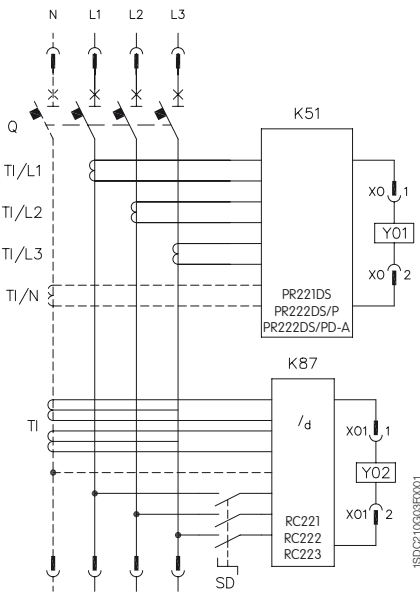
Disjoncteur tripolaire ou tétrapolaire avec déclencheur électronique PR221DS, PR222DS/P ou PR222DS/PD et bloc différentiel RC221, RC222 ou RC223 (uniquement tétrapolaire pour T4, T5 et T6)
