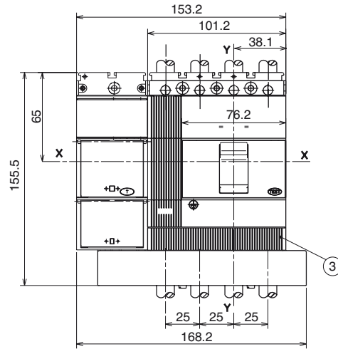
Prise avant - F
