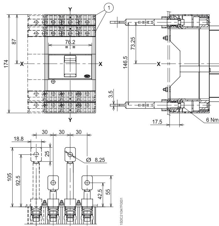
Arrière orientables - R
