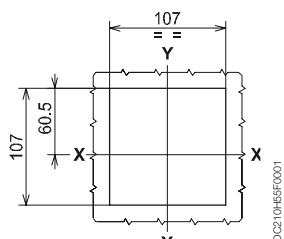
3-4 PÔLES Sans garniture
