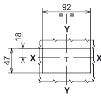
Sans garniture et disjoncteur en saillie (3 PÔLES)
