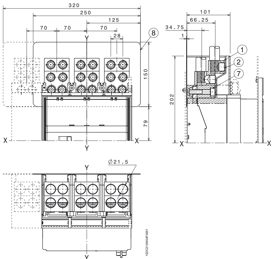
Avant pour câbles en cuivre/aluminium - FC CuAl 4x240 mm 2
