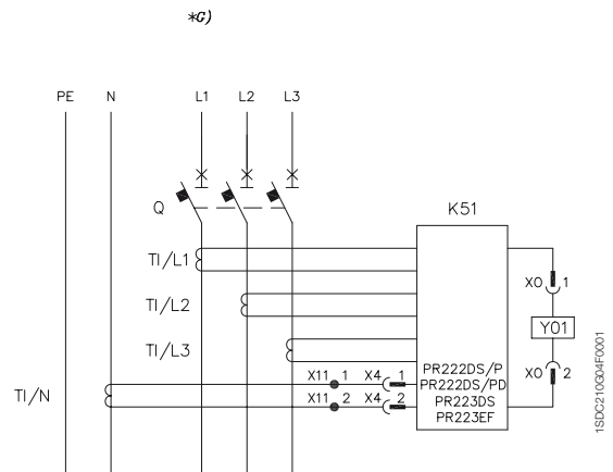
Disjoncteur tripolaire en version fixe avec transformateur de courant sur conducteur neutre extérieur au disjoncteur (pour T4, T5 et T6)
