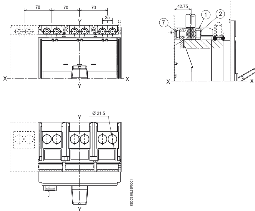
Avant pour câbles en cuivre/aluminium - FC CuAl 2x240 mm 2
