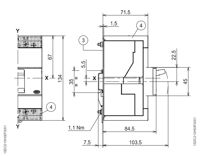
Fixation sur rail DIN EN 50022
