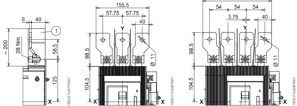
Avant prolongées épanouies 400 A - ES
