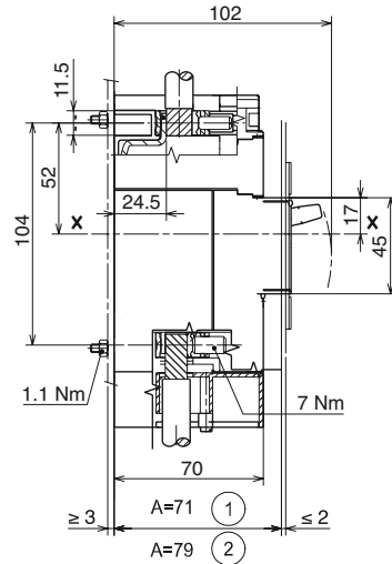
Fixation sur platine
