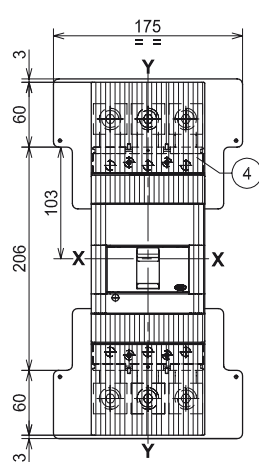
Avant pour câbles en cuivre/aluminium - FC CuAl 240 mm 2
