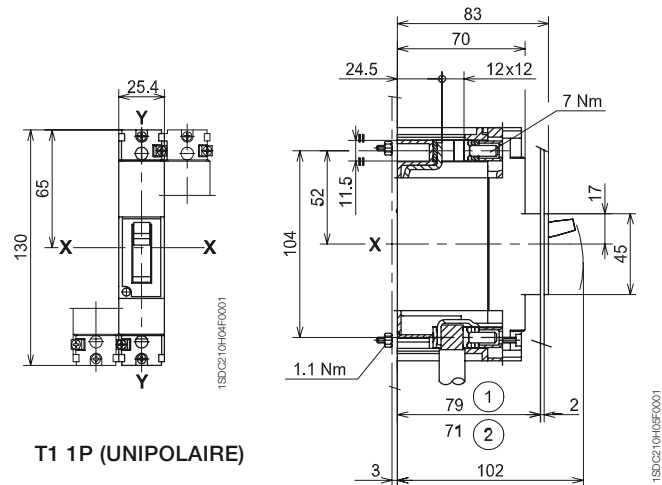
Disjoncteur sans blocs
