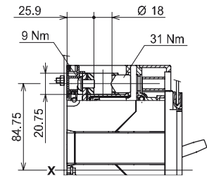
Avant pour câbles en cuivre/aluminium - FC CuAl
