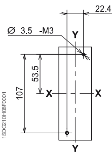
T1 1P (UNIPOLAIRE)
