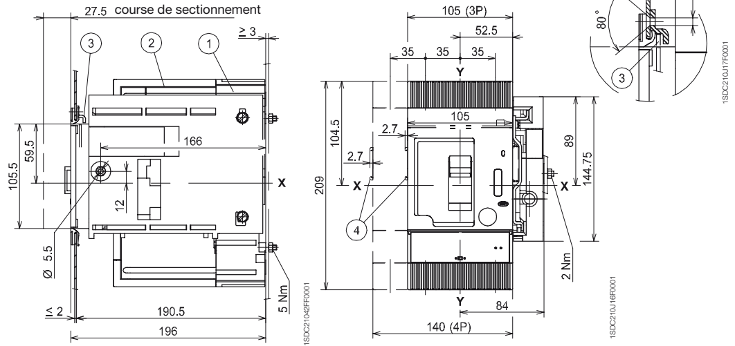
Fixation sur platine
