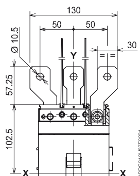
Avant prolongées épanouies - ES
