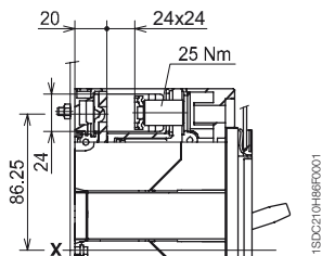
Avant pour câbles en cuivre - FC Cu
