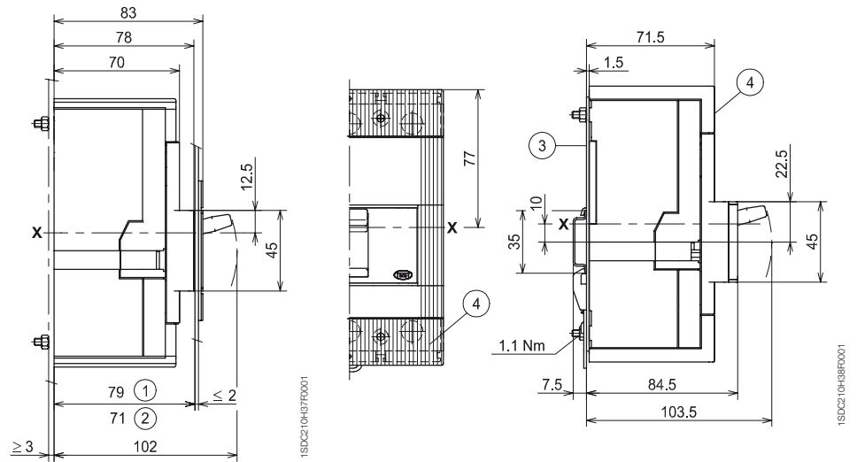
Fixation sur platine
