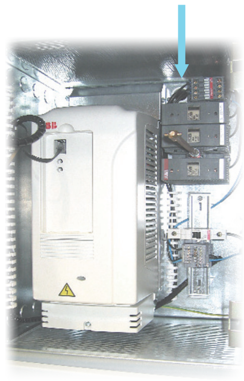
OS 隔离开关熔断器组
