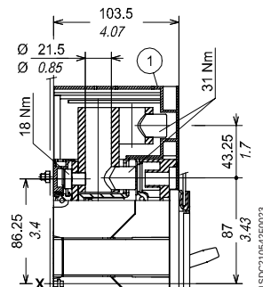
Front for copper/aluminium cables Cu/Al 2x240 mm 2 - FC CuAl
