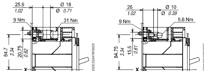
Front for copper/aluminium cables - FC CuAl
