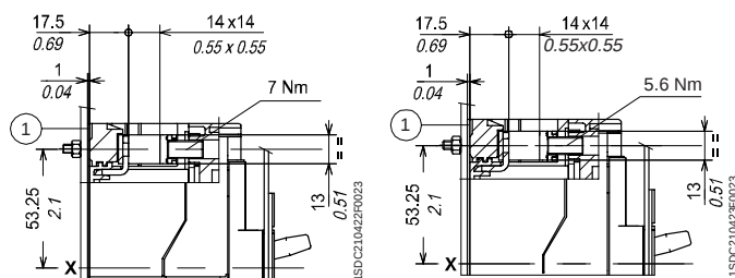
Front for copper/aluminium cables - FC CuAl 1/0 AWG/50 mm 2
