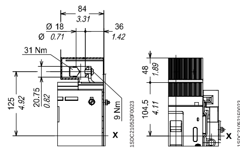
Front for copper/aluminium cables - FC CuAl
