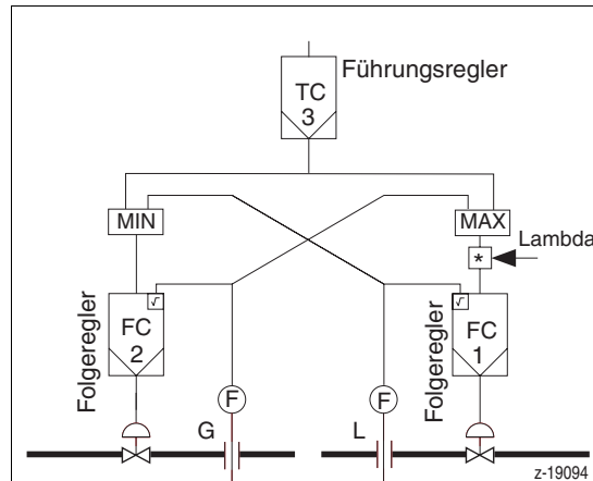
Bild 3-30 (z-19094) G = Gas L = Luft
