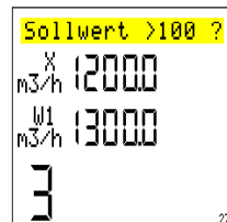
Bild 3-27 Beispiel: Loop 3 Temperaturregler Loop 2 Luftdurchflussregler Loop 1 Gasdurchflussregler
