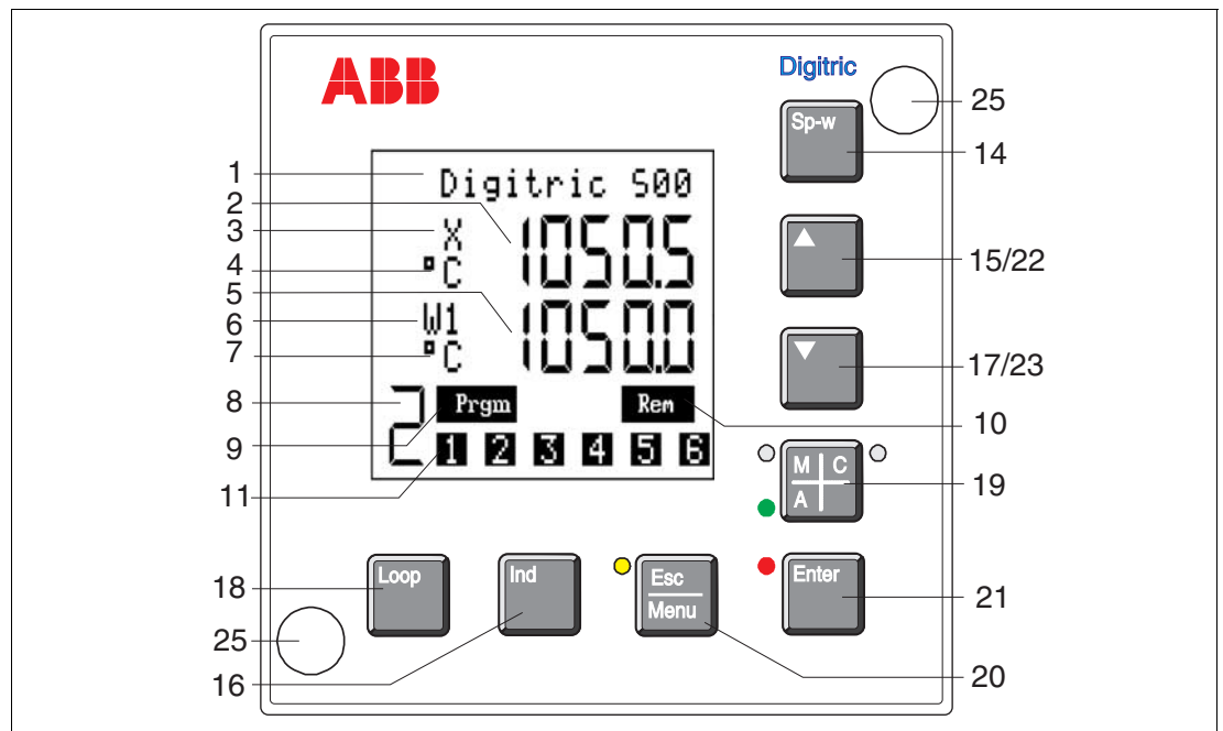
Bild 3-1 Gerätefront D500 (Digitric 500)
