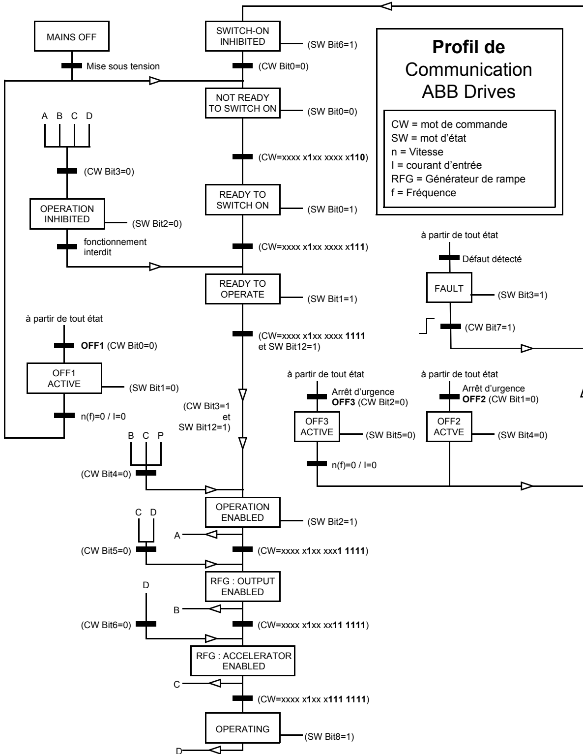
Figure 1 Séquentiel de commande du profil de communication ABB Drives.
