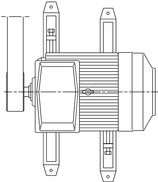
Figure 2. Glissières et entraînements à courroie
