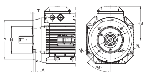
Flange-mounted motor, small flange; IM B14 (IM 3601)
