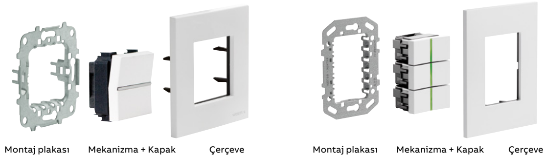
Montaj plakası
