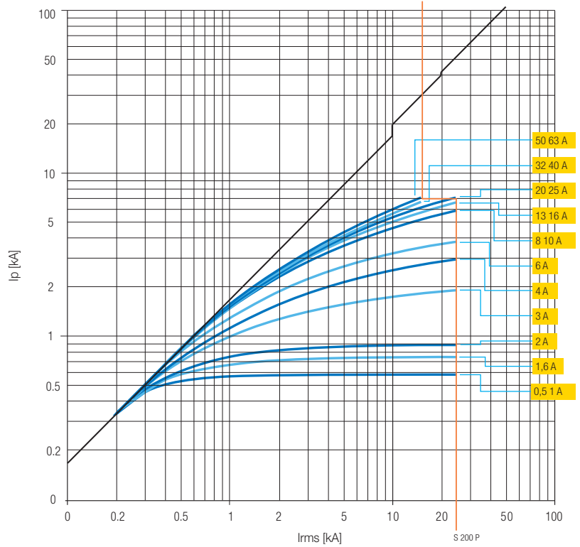
S 200 P, charakteristika Z
