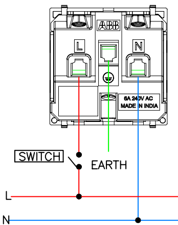
3+2 Pin socket
