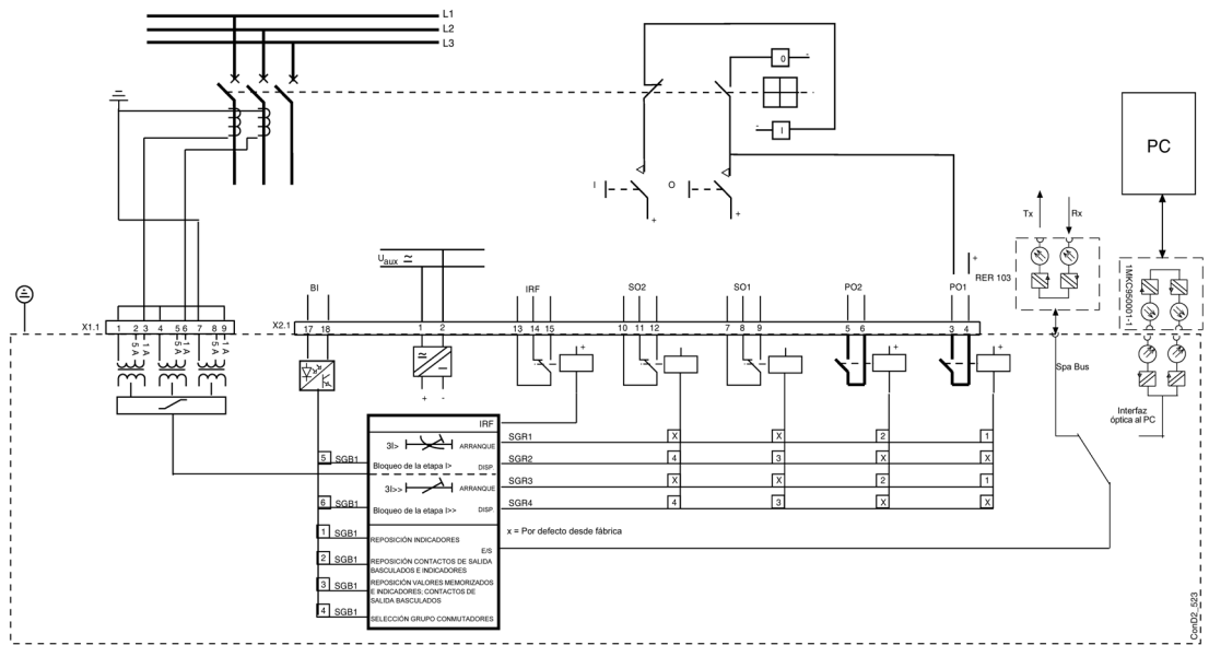
Fig. 2 Diagrama de conexión del relé de sobrecorriente
