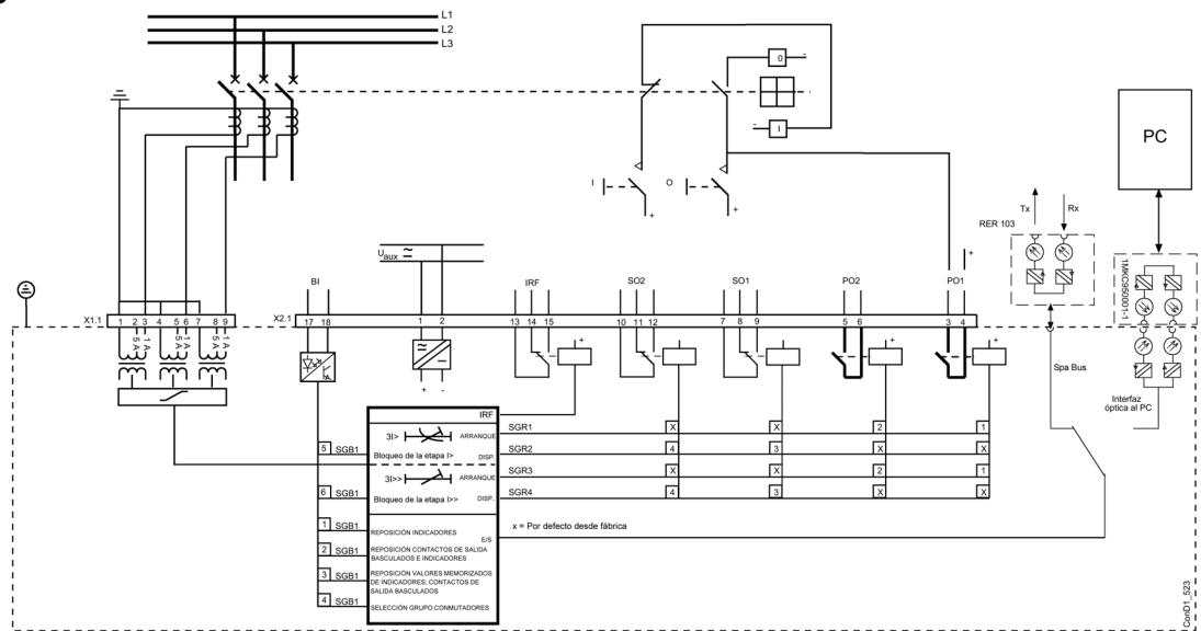
Fig. 1 Diagrama de conexión del relé de sobrecorriente
