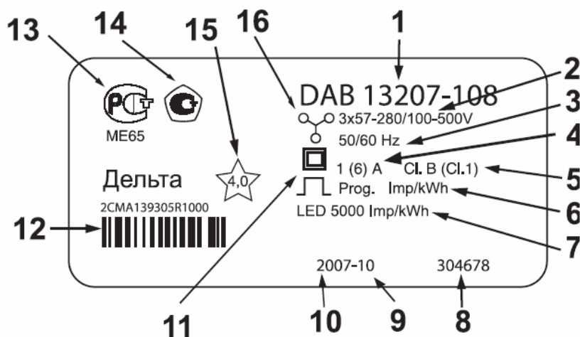
Рис. 2-2 Этикетка типа счетчика
