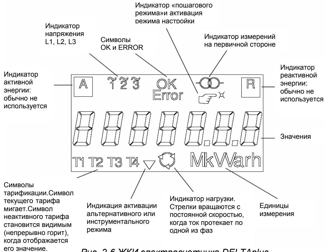
Рис. 2-6 ЖКИ электросчетчика DELTAplus
