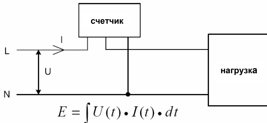
Рис. 5-4 Однофазные измерения
