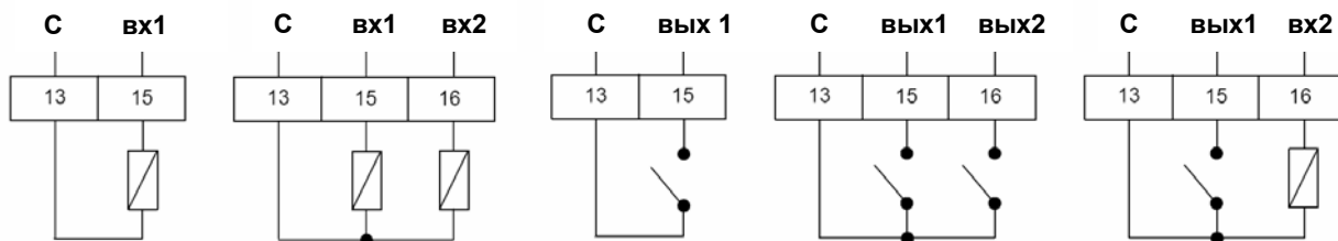
Рис. 4-7 Варианты входов/выходов
