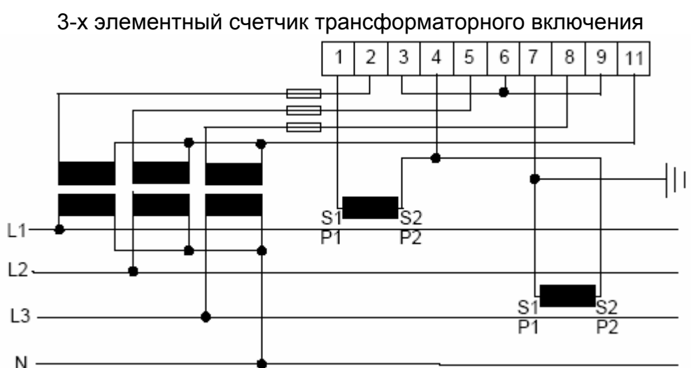
Рис. 5-13. Использование 3-х элементных счетчиков с 2 трансформаторами тока
