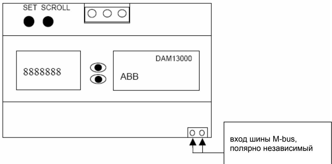
Рис. 6-2. Подключение к шине M-bus
