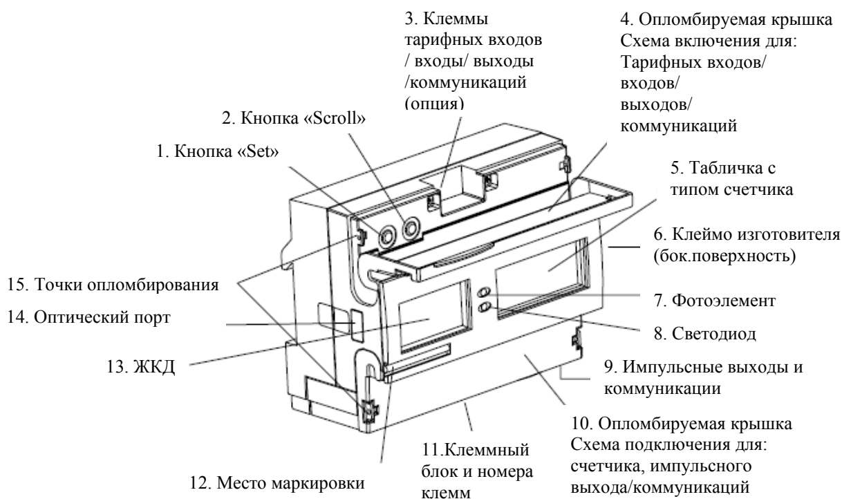
Рис. 2-1. Элементы электросчетчиков
