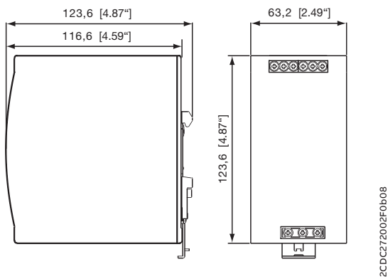
CP-E 24/5.0
