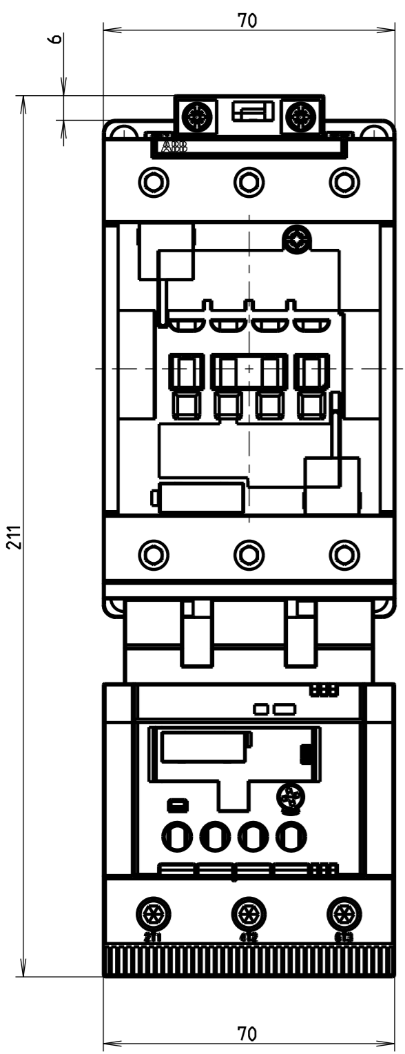
ECHELLE 1:2
